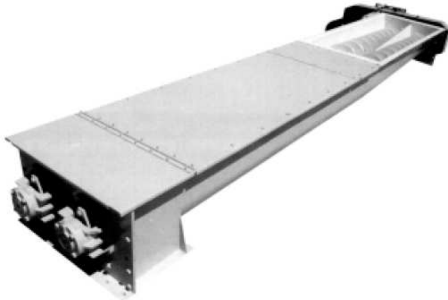
Obr. 20: Dvuhřídelový kónický šnekový odebírač fa HAS [12]
