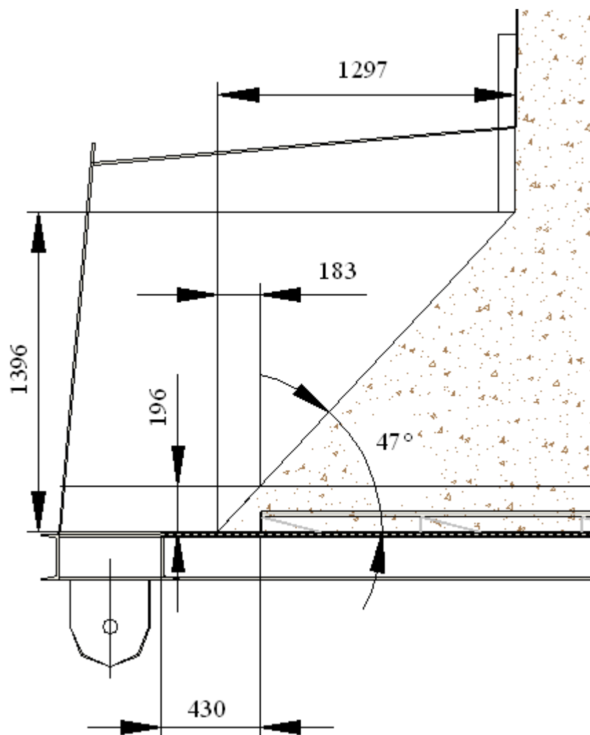
Obr. 31: Schéma vynášeného objemu hrablem
