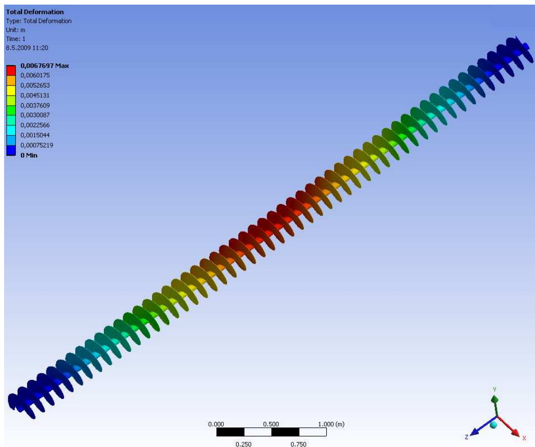
Obr. 36: Kontrola deformace šneku bez podpěrných ložisek v programu ANSYS
