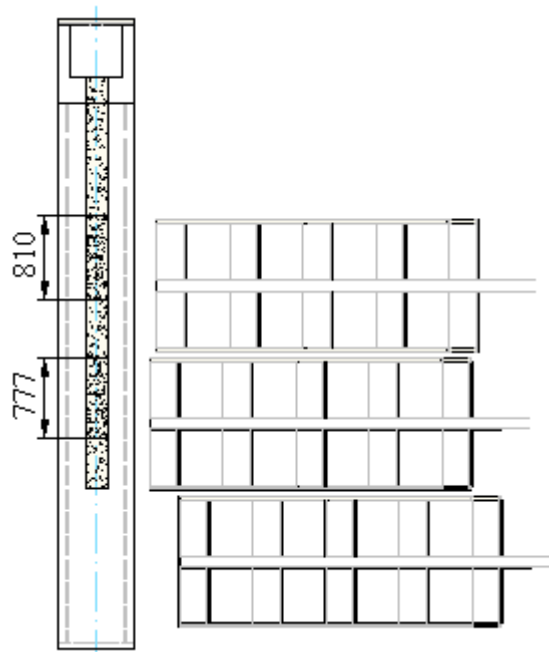
Obr. 47: Schéma vynášení materiálu v čase t = 47 s
