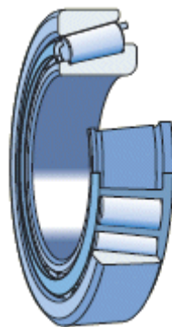
Obr. 41: Řez jednořadým kuželíkovým ložiskem
