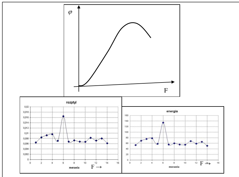
Obr.3 Tvar experimentálne nameranej závislosti pomerového kritéria optimality vrtania v závislosti na prítlaku (Sekula, 1992; Sekula et al., 1991) -hore; priebeh závislosti rozptylu a energie sprievodného akustického signálu na prítlaku pri vrtaní andezitu -dole.
