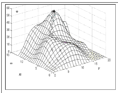
Obr.2 Predpokladaný tvar účelovej funkcie \varphi = \varphi(n, F) pre úlohu optimálneho riadenia procesu vŕtania.
