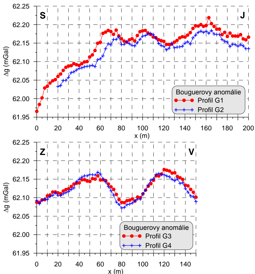
Obr.4 Gravimetrické měření na paralelních profilech G1, G2 a G3, G4.
