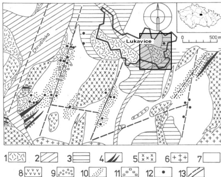
Obr.1 Geologické schéma okolí Lukavice u Chrudimi s vyznačením zájmového území se starými důlními díly. Legenda: 1- svahoviny, 2- aluvia, 3- křídové pískovce, 4- lamprofyrové žíly, 5- felsitické a granitové porfyry, 6- žumberecký granit, 7 – porfyroidy (kyselá metavulkanity), 8- „porfyroidy“ (bazické metavulkanity), 9 – silifikace, 10 – intenzivní argillitizace, 11 – pyritizace, 12 – významné vrty, 13- předpokládané a ověřené zlomy. Upraveno podle Jiránek a kol., (1993).
