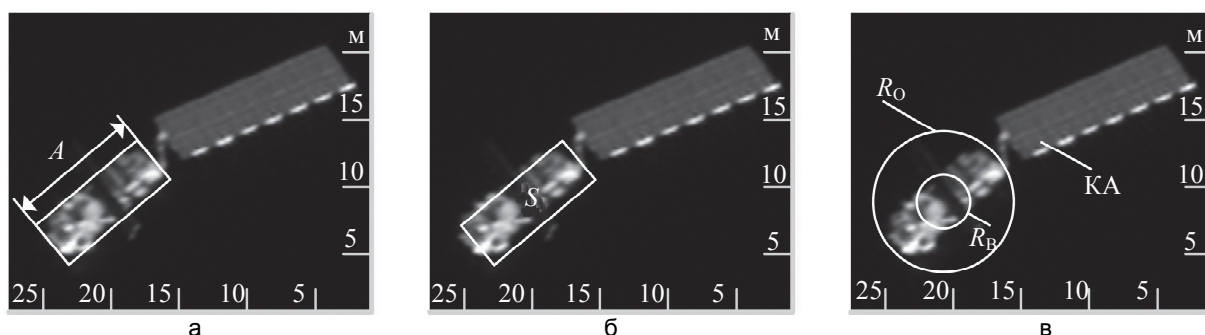
Рис. 2. К определению вероятности опознавания формы объекта: определение геометрического размера A объекта наблюдения по его изображению (а); определение площади S объекта наблюдения по его изображению (б); определение радиусов вписанной в контур R_B и описанной вокруг контура R_O объекта наблюдения окружностей по его изображению (в)
