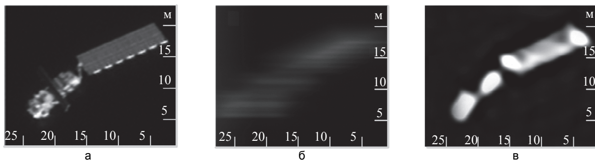
Рис. 1. Результаты моделирования космического снимка аварийного спутника «ENVISAT»: изображение пригодное для обработки (а); «смазанное» изображение (б); изображение с низким пространственным разрешением (в)
