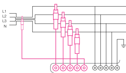
Sistema Trifàsic 4 fils
