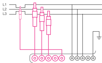
Sistema Trifàsic 3 fils
