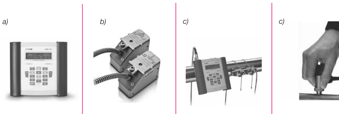
Figura 11.14. Cabalímetre + accessoris
