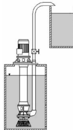
Figura 11.10. Esquema del bombeig d'un fluid mitjançant una bomba centrífuga vertical.
