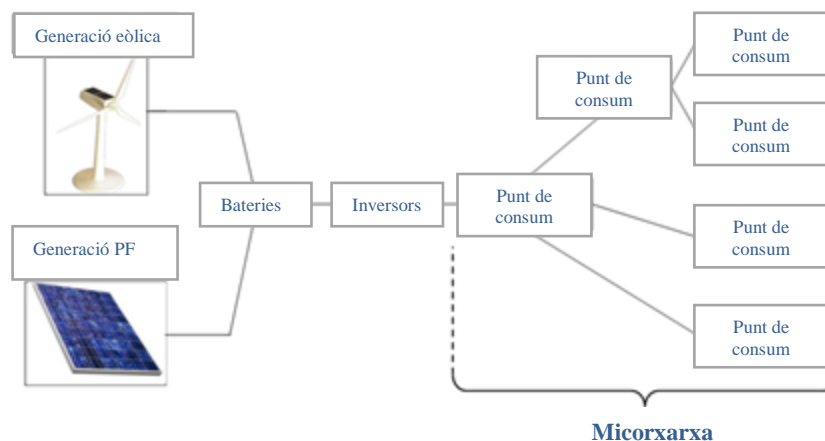
Figura 2.1 – Esquema d'un sistema d'electrificació rural autònoma d'una única microxarxa [Ferrer-Martí et al. , 2013]
