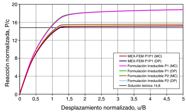
Figura 6. Curva Desplazamiento-Reacción.
