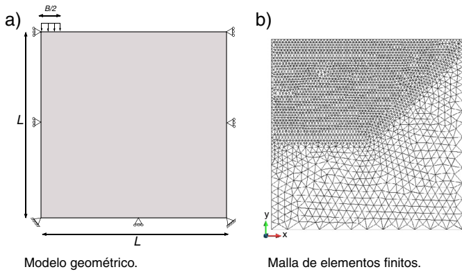
Figura 4. Geometría y malla empleada en el ensayo de Prantl.
