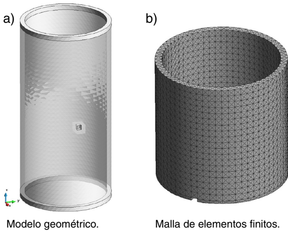
Figura 12. Geometría y malla empleada.
