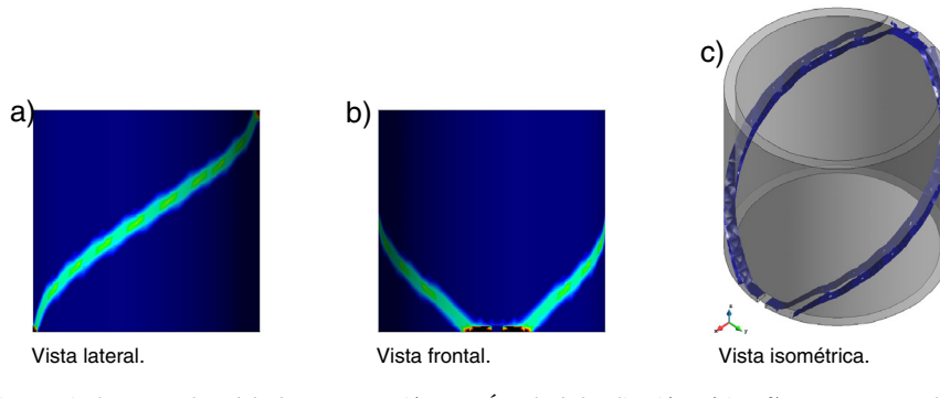
Figura 13. Deformaciones plásticas equivalentes en el modelo de VM en tracción pura. Ángulo de localización teórico: \theta_{loc}^{teo} = \pm 45.0^\circ con el eje vertical. Ángulo de localización numérico: \theta_{loc}^{num} = \pm 45.0^\circ .
