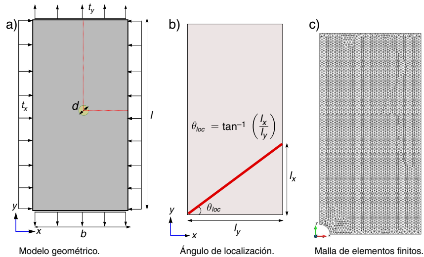
Figura 7. Geometría y malla empleada.
