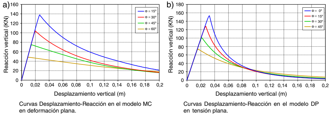
Figura 11. Curvas Desplazamiento-Reacción.
