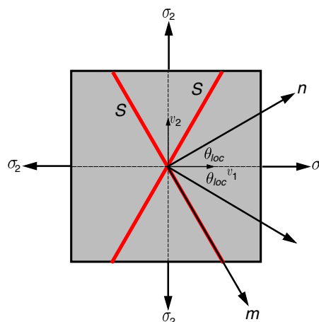
Figura 3. Ángulo de localización.
