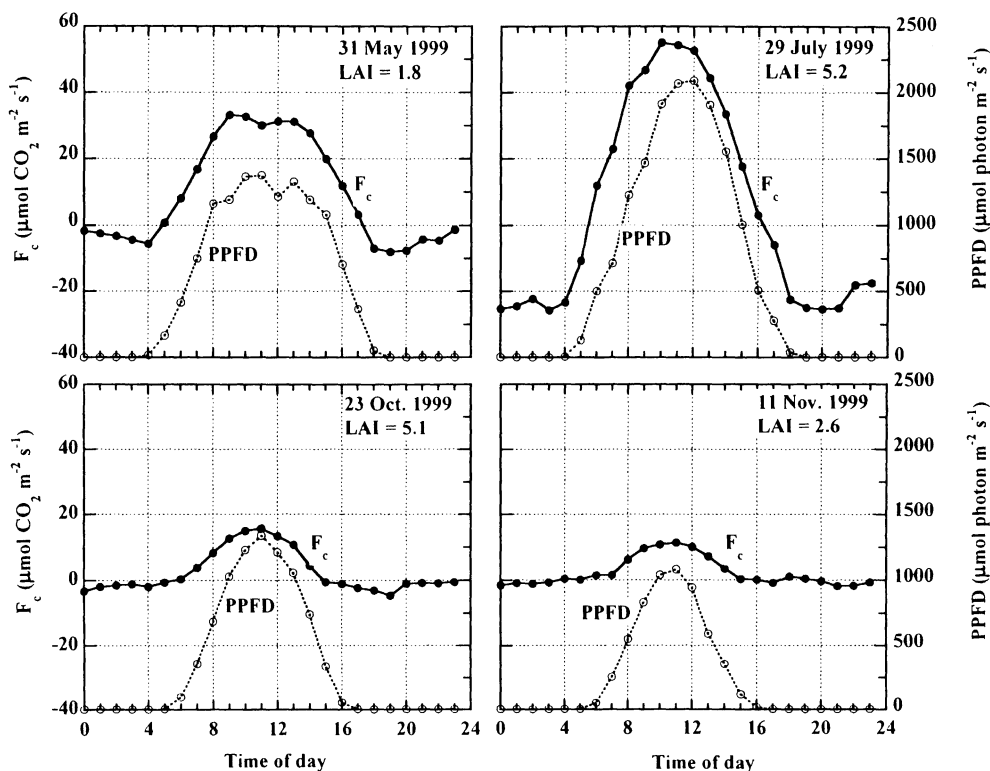
図1 1時間ごとのCO 2 フラックス( F_c )と光合成有効光量子密度(PPFD)の日変化
