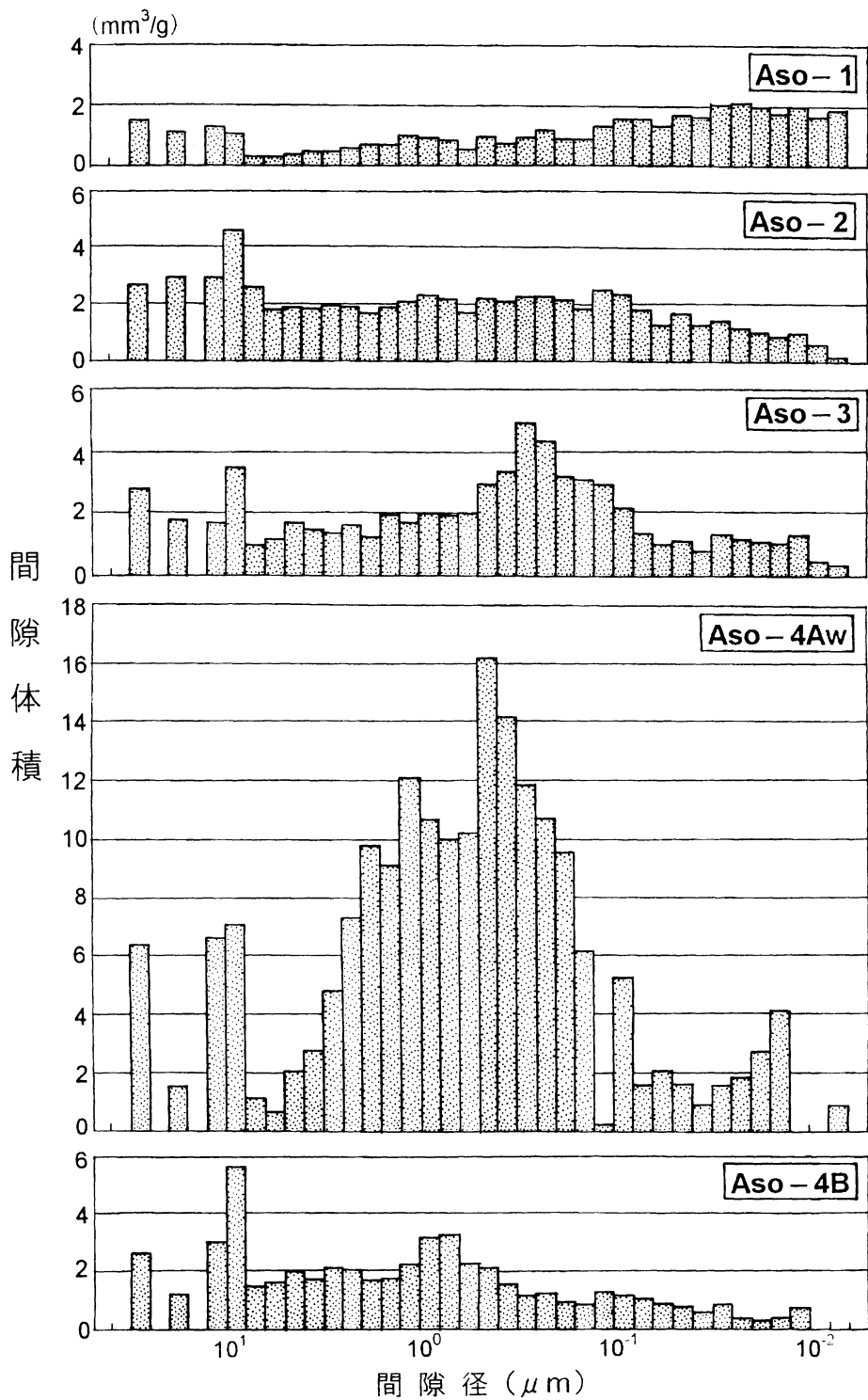
第1図 阿蘇火砕流堆積物(熔結凝灰岩)の間隙径分布
