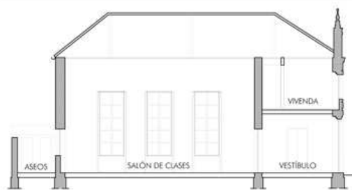
SECCIÓN LONXITUDINAL
