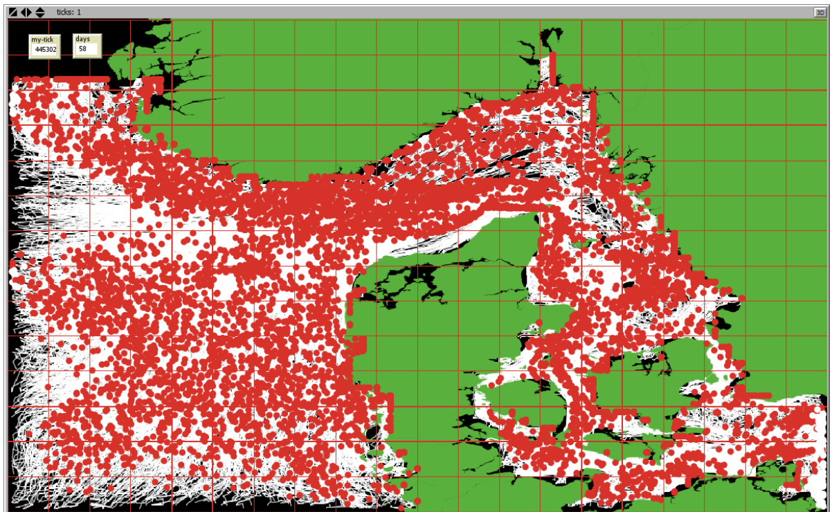
Figur 3. Slutpositioner af agenter (røde prikker) og agent-spor (hvide liner) fra en spredningsberegning foretaget med SRAAM-værktøjet, baseret på 2 måneders simuleringsperiode og knap 10 000 agenter. Det hydrografiske datagrundlag er HBM modellen som leveres af DMI. Landområder er angivet med grønt. Simuleringen er kørt med agenter med en varighed af det pelagiske stadie på 30 dage. De røde linjer i et kvadratisk net, repræsenterer inddeling af modelområdet i et regulært grid af delområder, for hvilket der er konstrueret en sammenhængsmatrix, der beskriver sandsynligheden for at agenter der tilføres/udledes i et delområde ender med at settle i et af de øvrige delområder.
