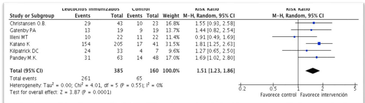
Figura 4. Forest plot recién nacido vivo.
