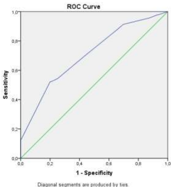
Ilustración 51. Curva ROC para discriminación del modelo
