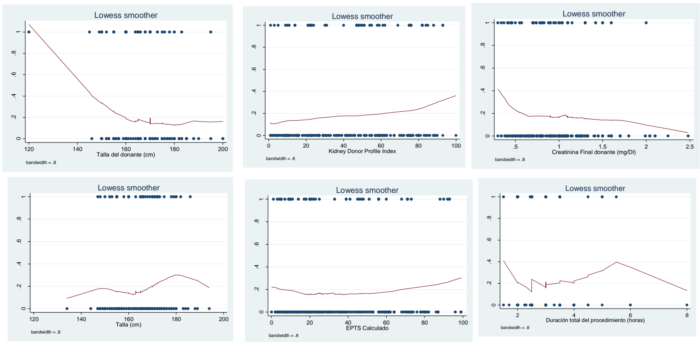
Ilustración 36. Gráficas de monotonía para variables cuantitativas- STATA®.
