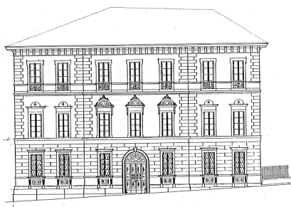
Südfassade
