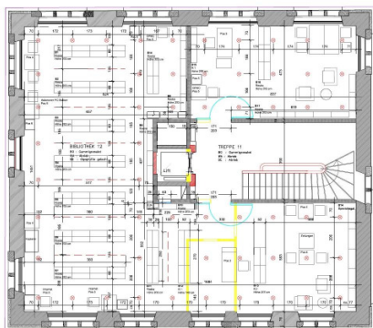
1. Obergeschoss
