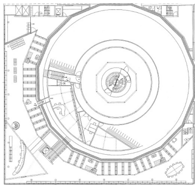
1. Obergeschoss
