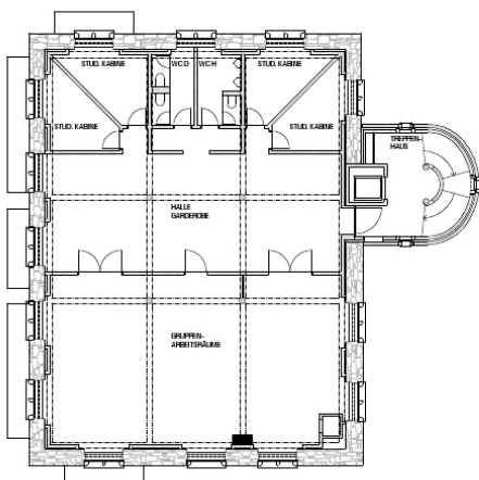
3. Obergeschoss
