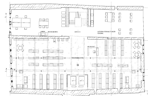
3. Obergeschoss
