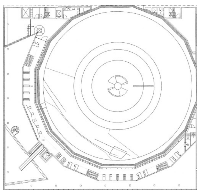
3. Obergeschoss
