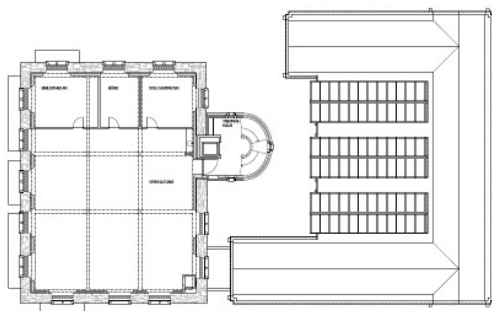
2. Obergeschoss
