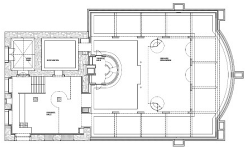
Erdgeschoss
