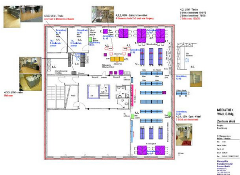
2. Obergeschoss, ODIS
