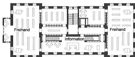
1. Obergeschoss
