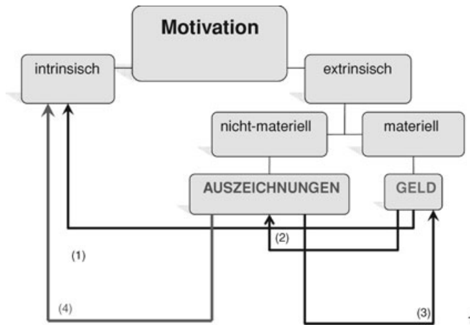
Abbildung 1 Einige Wirkungszusammenhänge
