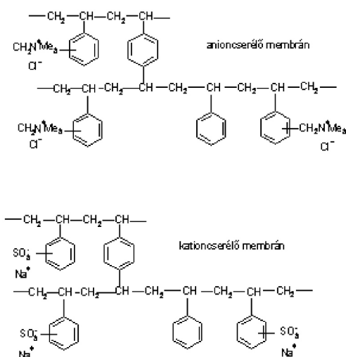
1. Ábra. Anion- és kationcserélő membránok felépítése
