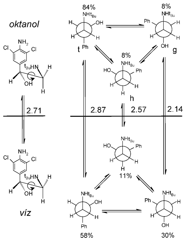
7. ábra. A klenbuterol és rotamerjeinek megoszlási sémája a rotamerok százalékos eloszlásával és a klenbuterol egészének, valamint az egyes rotamerok megoszlási hányadosának a log értékeivel.
