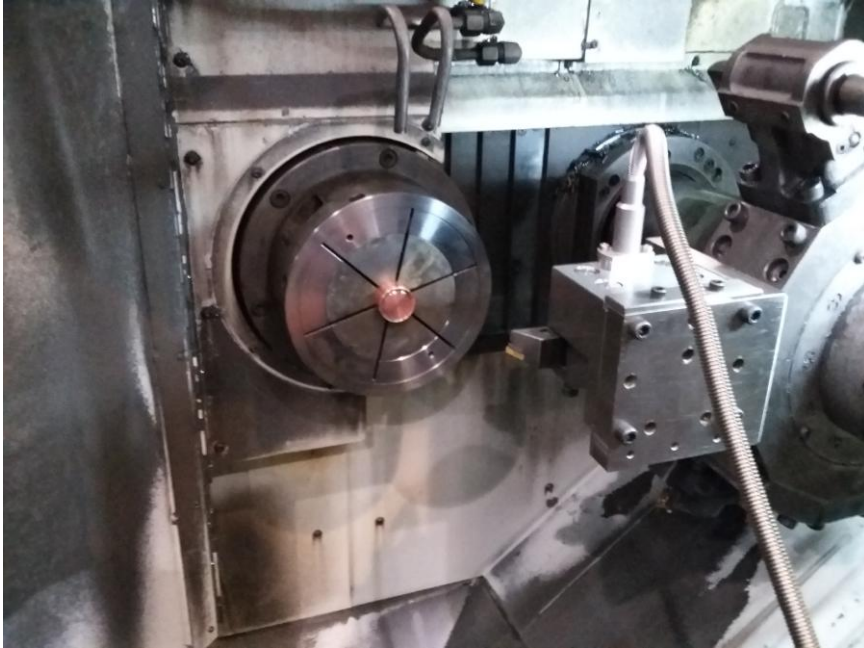
Resim 1. Kesme Kuvveti Ölçme Düzeneği
