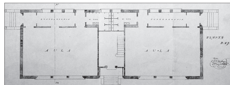
Plànol de la planta baixa.
