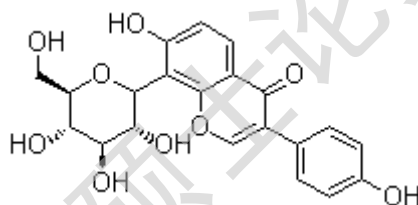
图 3 PU 的结构式
