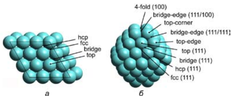
Рис. 1. Центры адсорбции поверхности Pt(111) (а) и нанокластера \text{Pt}_{79} (б)
