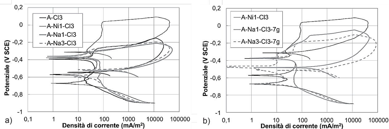
Fig. 2 – Prove potenziodinamiche effettuate in soluzione alcalina in presenza di cloruri 0,3 mol/L aggiunti immediatamente (a) o, solo nel caso del nitrato, dopo una settimana di permanenza del campione in soluzione alcalina inibita (b) – Potentiodynamic polarization in alkaline solution in presence of 0.3 mol/L chlorides added immediately (a) or, only for nitrate, after 1 week of sample immersion in inhibited alkaline solution (b)
