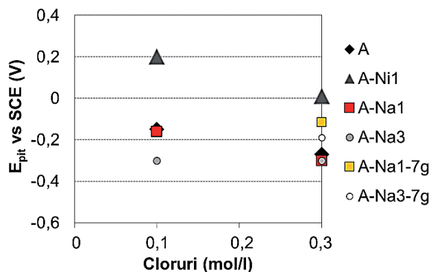
Fig. 3 – Potenziale di pitting risultante dalle prove di polarizzazione potenziodinamica, in funzione della presenza di inibitori e del contenuto di cloruri – Pitting potential resulting from potentiodynamic polarization tests, as a function of the presence of inhibitors and chlorides
