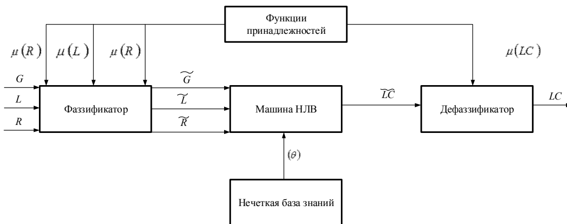
Рис. 1 – Система НЛВ, реализующая принятие решений по выбору маршрута доставки ЖРК на металлургические предприятия Мариуполя
