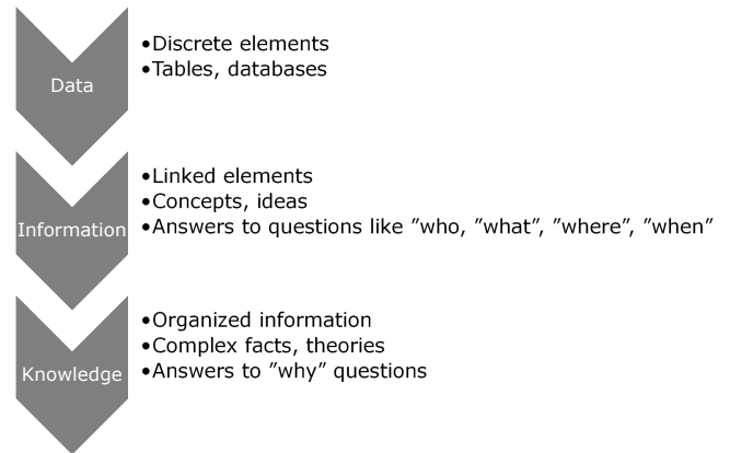
Fig. 3. DIKW Diagram.
