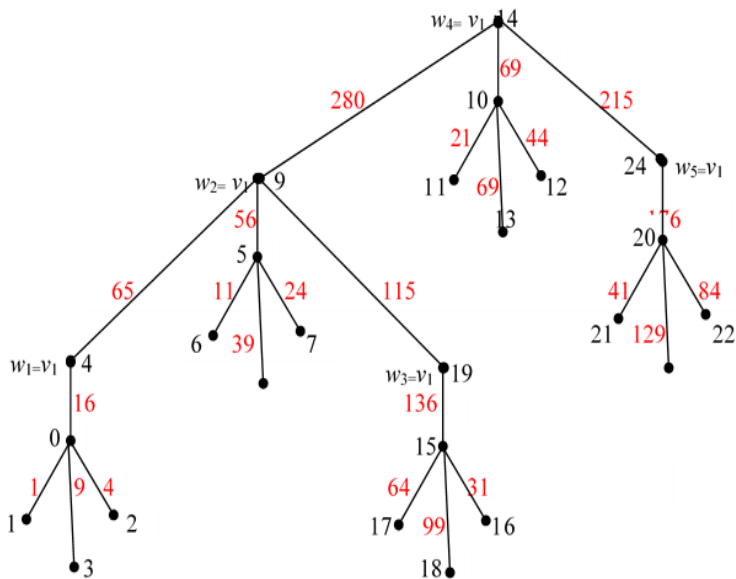
Рис. 3. Квадратная разностная разметка дерева \Delta T
