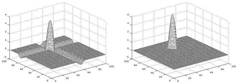
Рис.2. МНК (слева) и МНМ (справа) для регулярной 3D-структуры с одним дефектом
