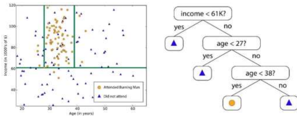
Kuva 5. Päättöpuun toimintaperiaate (Microsoft 2017a)
