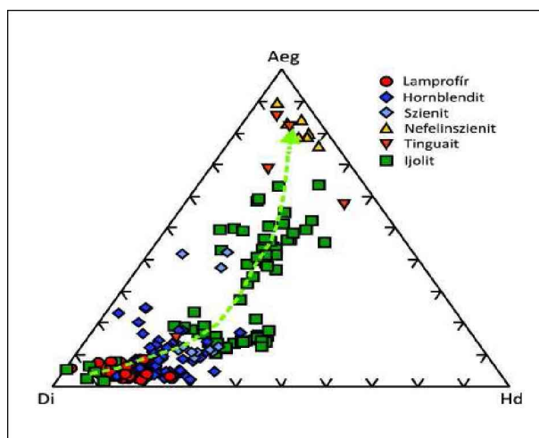
2. ábra – Klinopiroxének Di-Hd-Aeg (mol%) összetétele a Ditrói Alkáli Masszívum közeteiben
