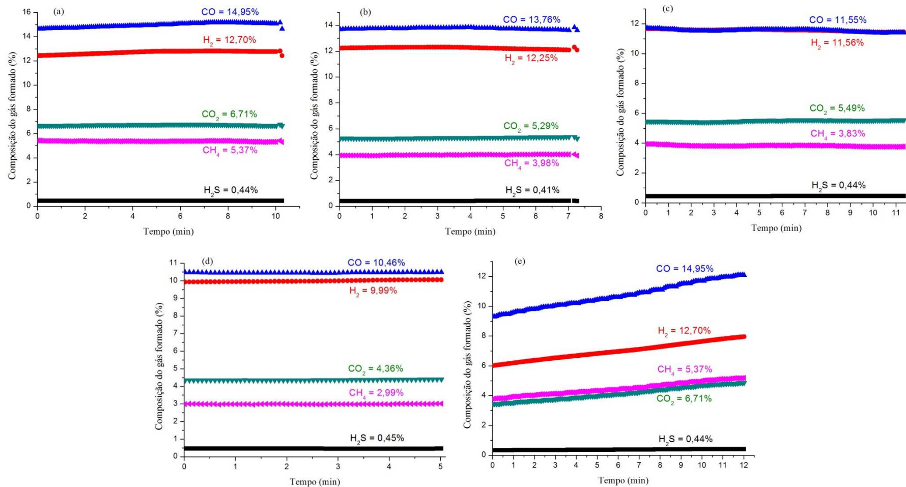
Figura 8.13 - Perfis de composição percentual dos de gases formados no processo de produção de gás combustível de Eucalyptus grandis com nitrogênio para (a) 12 NL/min (b) 14 NL/min (c) 16 NL/min (d) 18 NL/min.
