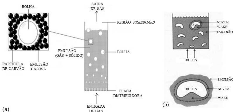
Figura 3.9 – (a) Representação das fases bolha e emulsão que constituem o leito fluidizado. 33 (b) Representação das fases bolha, emulsão, nuvem e wake. 34
