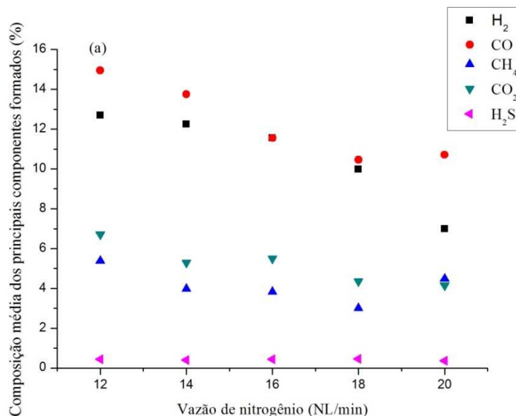
Figura 8.14 - Perfis de formação média (em porcentagem) de gases no processo de gaseificação de Eucalyptus grandis utilizando ar como agente de fluidização.
