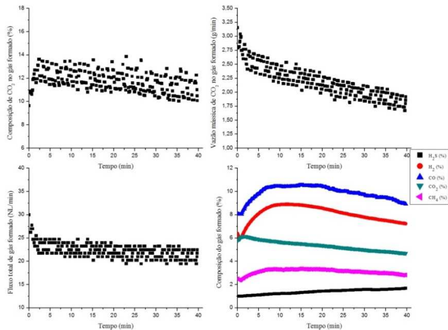
Figura 12.17 - Perfis do gás \text{CO}_2 em porcentagem e vazão mássica (g/min), fluxo total volumétrico de gás formado (NL/min), e composição do gás formado determinado no analisador de gases considerando a injeção de \text{N}_2 (%), em função do tempo, em gaseificação utilizando vapor como agente de fluidização para \text{SBR} = 3,10 .
