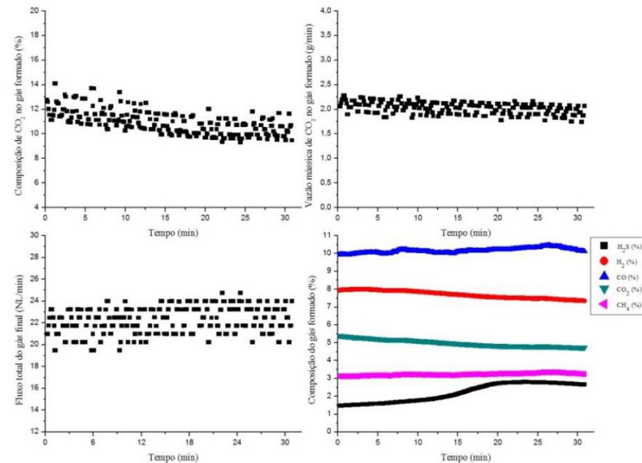
Figura 12.20 - Perfis do gás CO 2 em porcentagem e vazão mássica (g/min), fluxo total volumétrico de gás formado (NL/min), e composição do gás formado determinado no analisador de gases considerando a injeção de N 2 (%), em função do tempo, em gaseificação utilizando vapor como agente de fluidização para SBR = 3,38.
