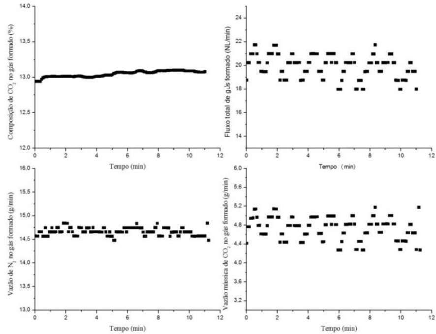
Figura 11.17 - Perfil do gás \text{CO}_2 em porcentagem, fluxo total volumétrico de gás formado (NL/min), e vazão mássica de \text{N}_2 e \text{CO}_2 em função do tempo em gaseificação utilizando ar como agente de fluidização para \text{RE} = 0,40 .
