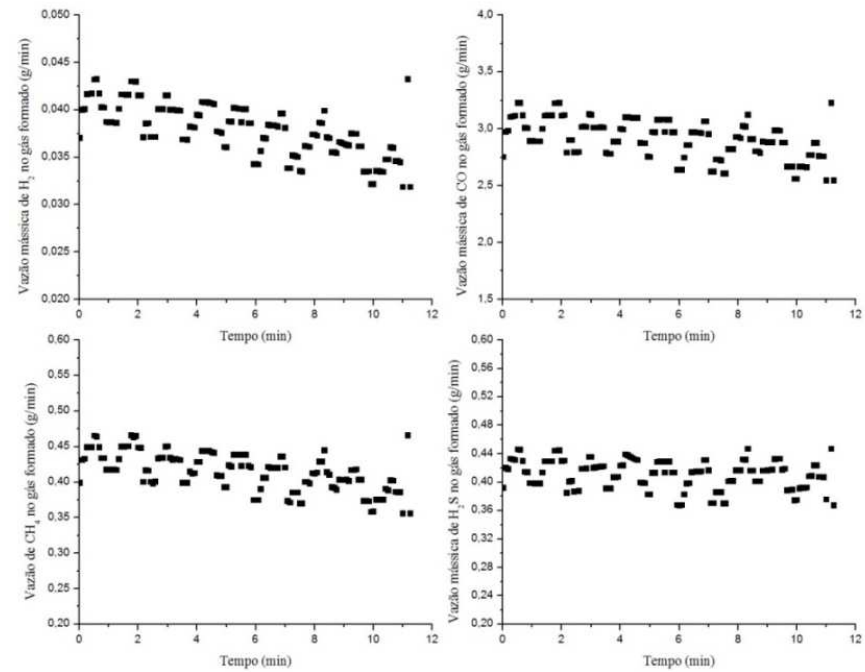
Figura 11.18 - Perfis de vazão (g/min) dos gases \text{H}_2 , \text{CO} , \text{CH}_4 e \text{H}_2\text{S} , em função do tempo, formados em gaseificação utilizando ar como agente de fluidização para \text{RE} = 0,40 .
