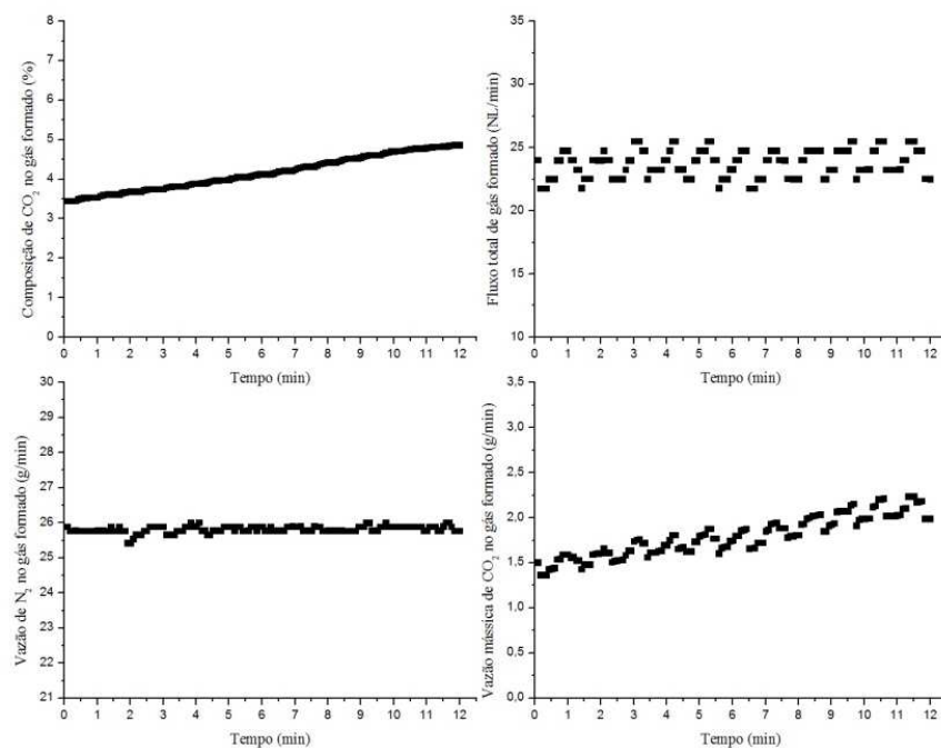
Figura 13.14 - Perfis do gás CO 2 em porcentagem e vazão mássica (g/min), fluxo total volumétrico de gás formado (NL/min), e vazão volumétrica de nitrogênio de entrada (NL/min), em pirólise utilizando 20 NL/min de nitrogênio como agente de fluidização.
