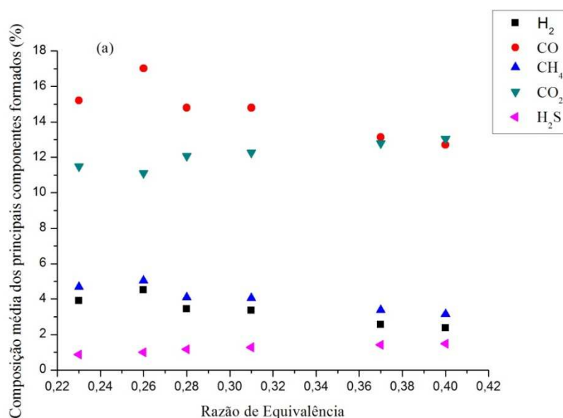
Figura 8.6 – Perfis de formação média (em porcentagem) de gases no processo de gaseificação de Eucalyptus grandis utilizando ar como agente de gaseificação.
