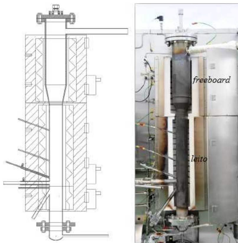
Figura 5.4 – Sistema de reação em leito fluidizado. 48
