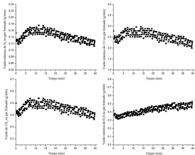
Figura 12.18 - Perfis de vazão (g/min) dos gases \text{H}_2 , \text{CO} , \text{CH}_4 e \text{H}_2\text{S} , em função do tempo, formados em gaseificação utilizando vapor como agente de fluidização para \text{SBR} = 3,10 .
