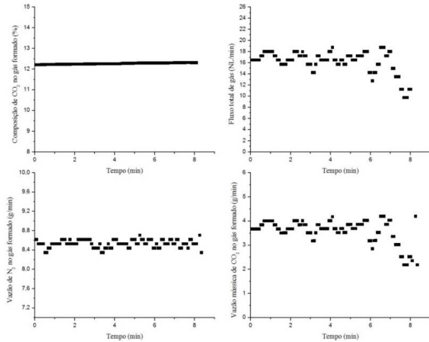
Figura 11.11 - Perfil do gás CO 2 em porcentagem, fluxo total volumétrico de gás formado (NL/min), e vazão mássica de N 2 e CO 2 em função do tempo em gaseificação utilizando ar como agente de fluidização para RE = 0,31
