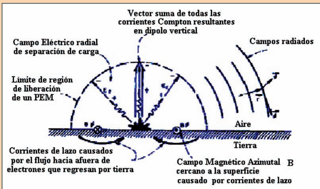
Figura 3 .- Radiación de un pulso electromagnético (PEM) a través de una antena vertical en tierra.
