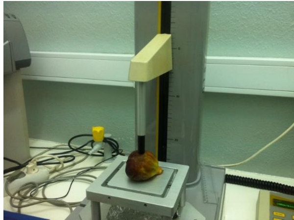
Figura 1 – Ensaio de Compressão/penetração a um Figo.
