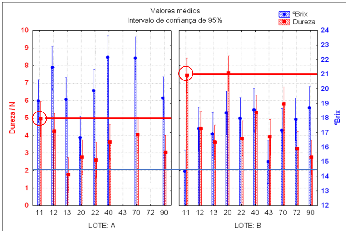
Figura 8 – Valores médios de dureza e de ^{\circ} Brix para as diferentes modalidades de amostra dos figos.
