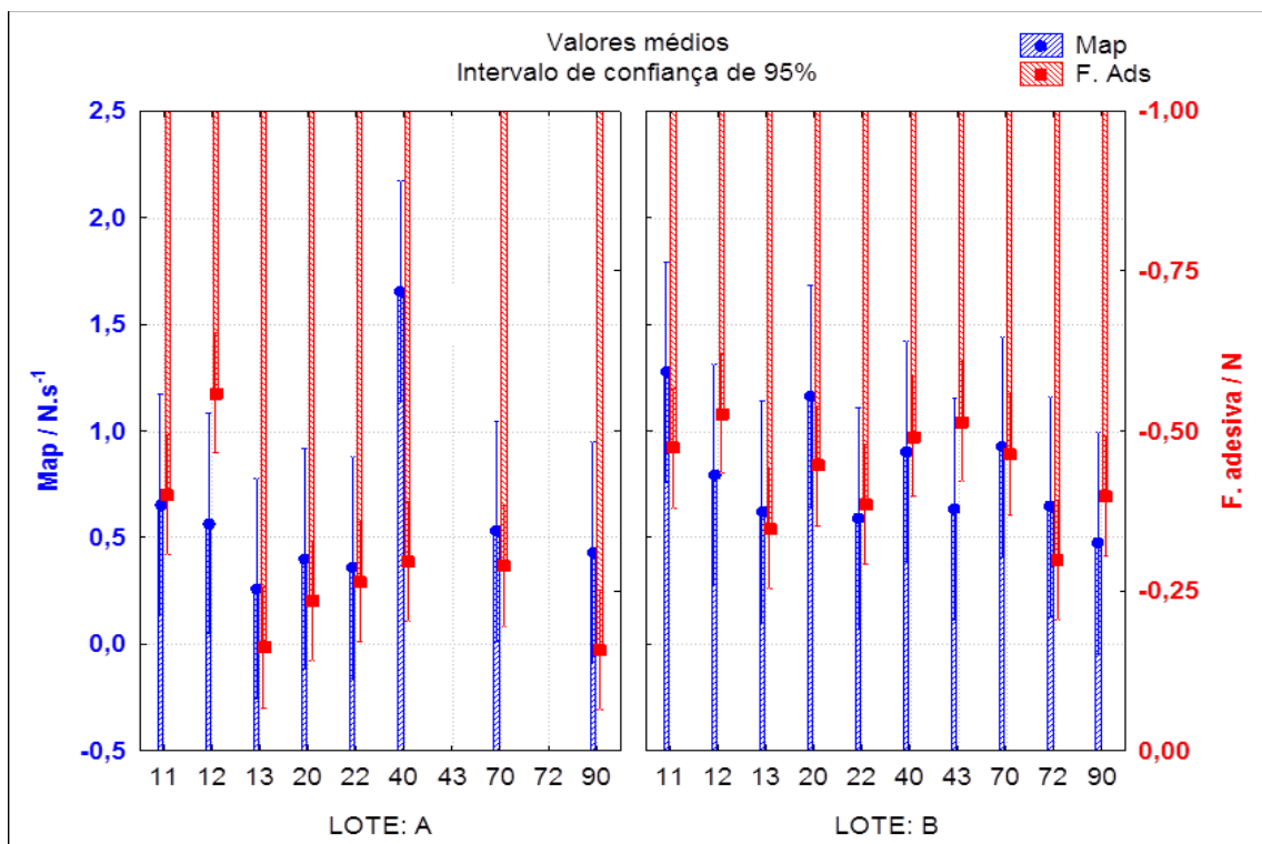
Figura 9 – Valores médios de força adesiva e módulo aparente para as diferentes modalidades de amostra dos figos.
