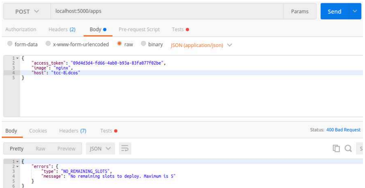
Figura 16 - Execução da aplicação sendo recusada devido ao limite de aplicações do usuário
