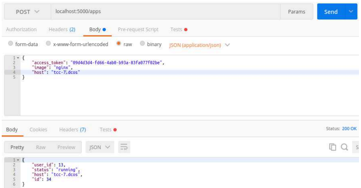
Figura 15 - Aplicação executando com sucesso para o host informado
