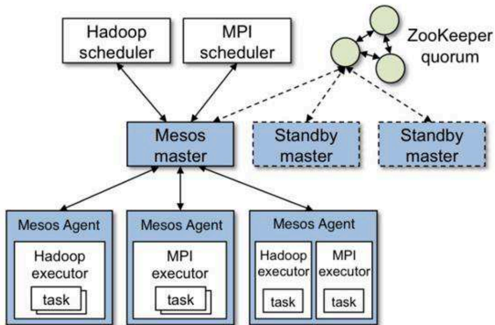
Figura 5: arquitetura básica do Mesos
