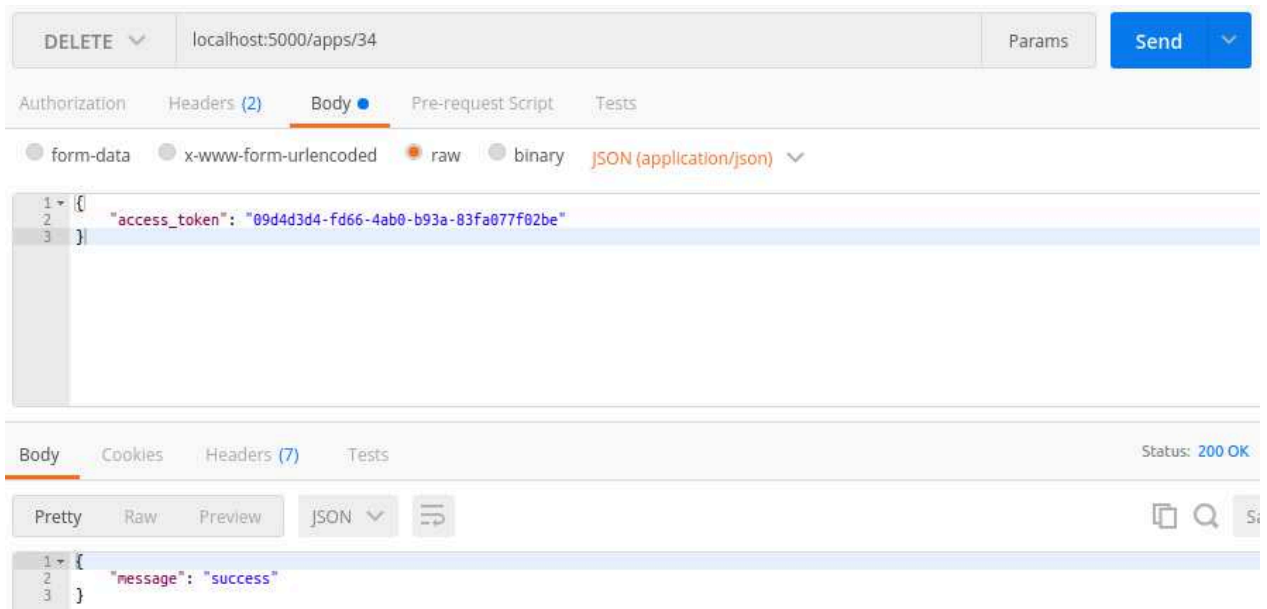
Figura 17 - Remoção de uma aplicação
