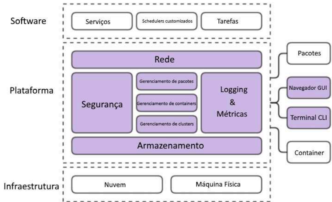
Figura 4. Camadas de arquitetura do DC/OS
