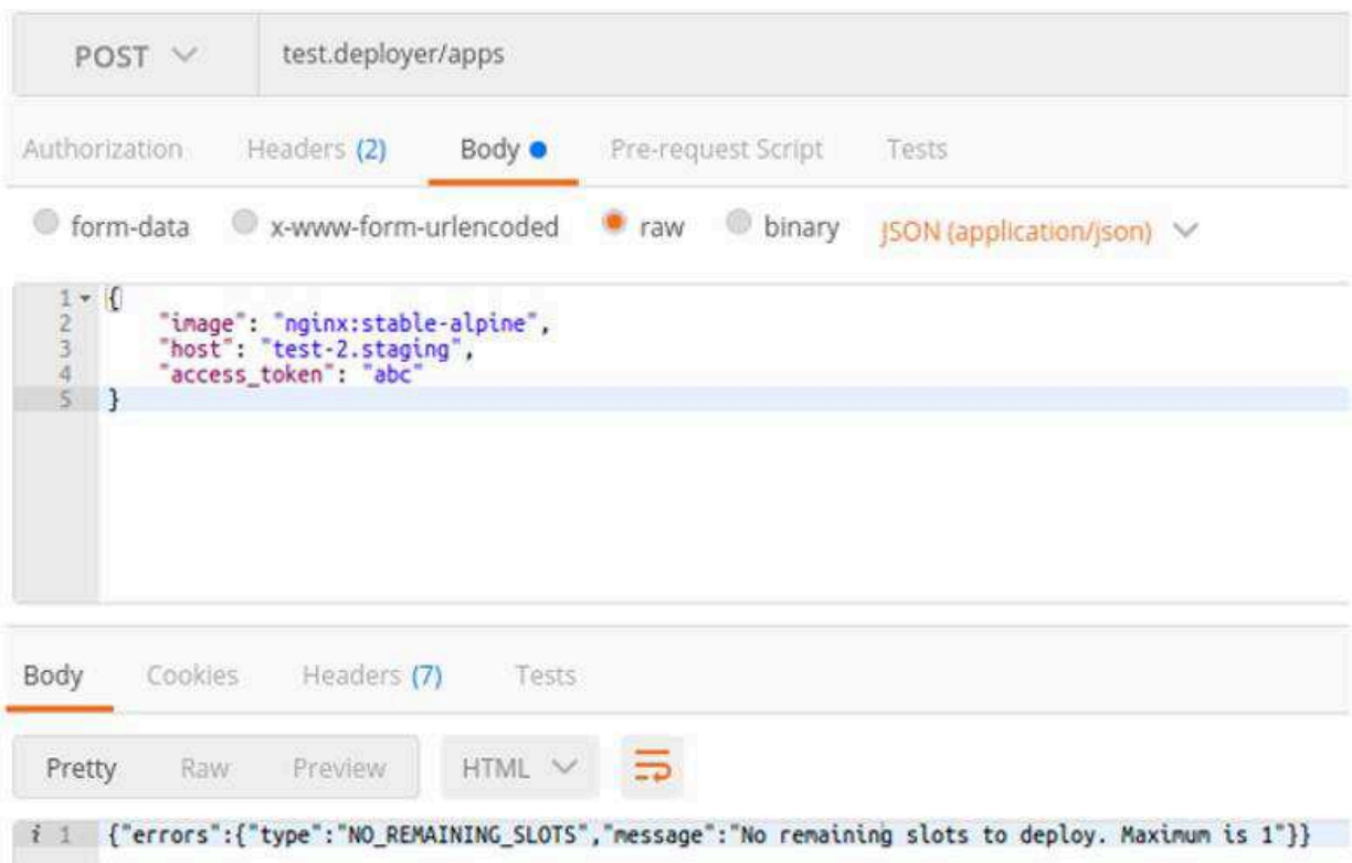
Figura 21 - Erro de um usuário tentando executar mais aplicações que seu limite permitido
