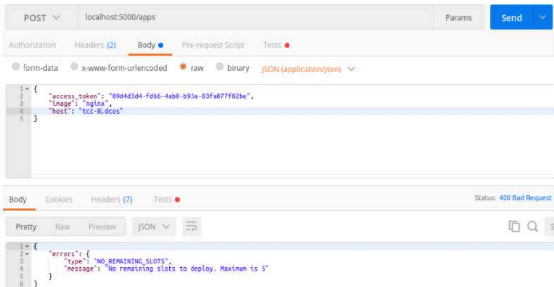
Figura 8. EndPoint POST/apps rejeitando deploy por exceder o limite
