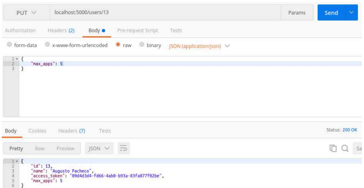
Figura 12 - Atualização de um usuário
