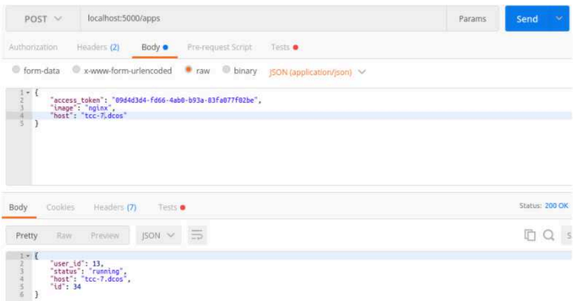
Figura 9. EndPoint POST/apps realizando um deploy com sucesso
