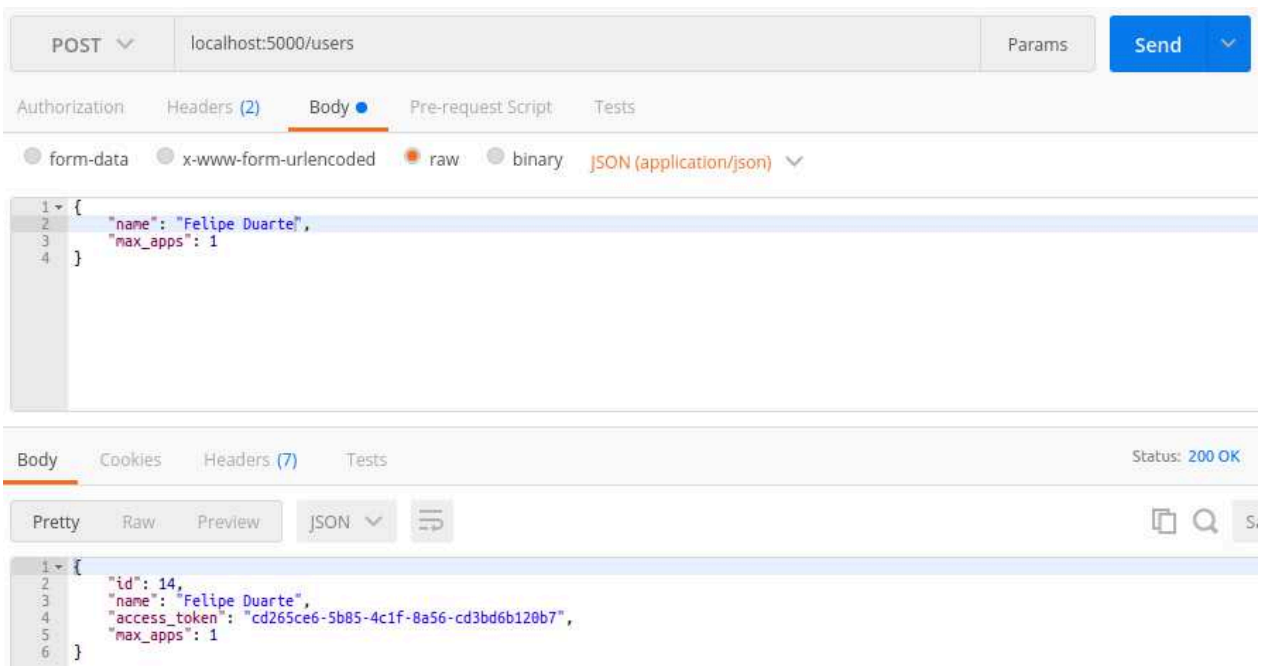
Figura 11 - Criação de um usuário na ferramenta
