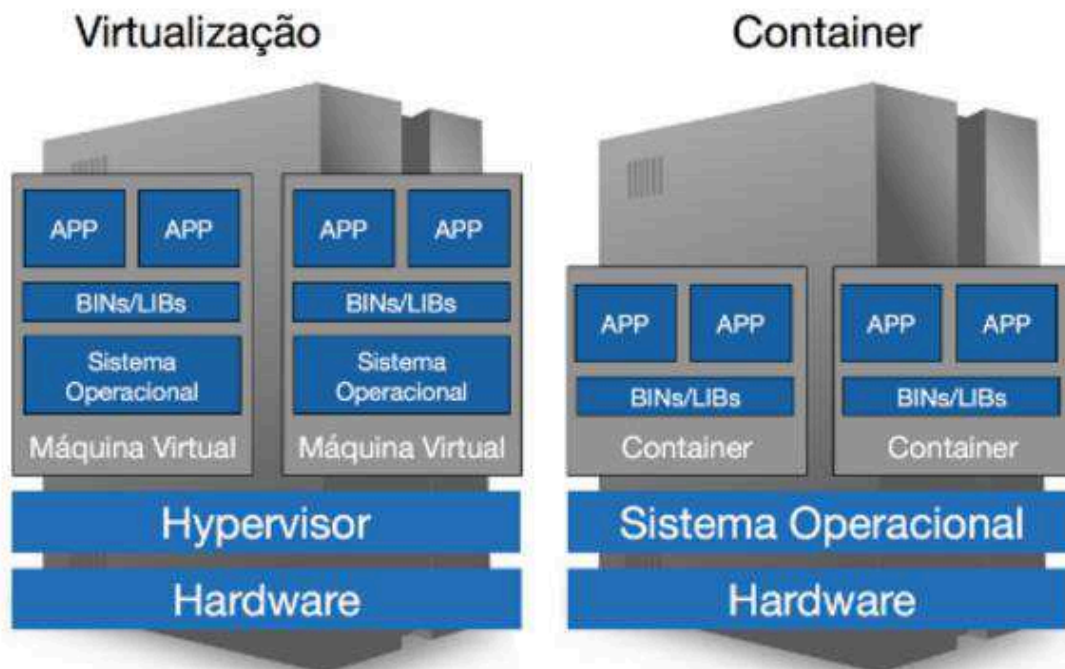
Figura 1: comparação Container x Virtualização
