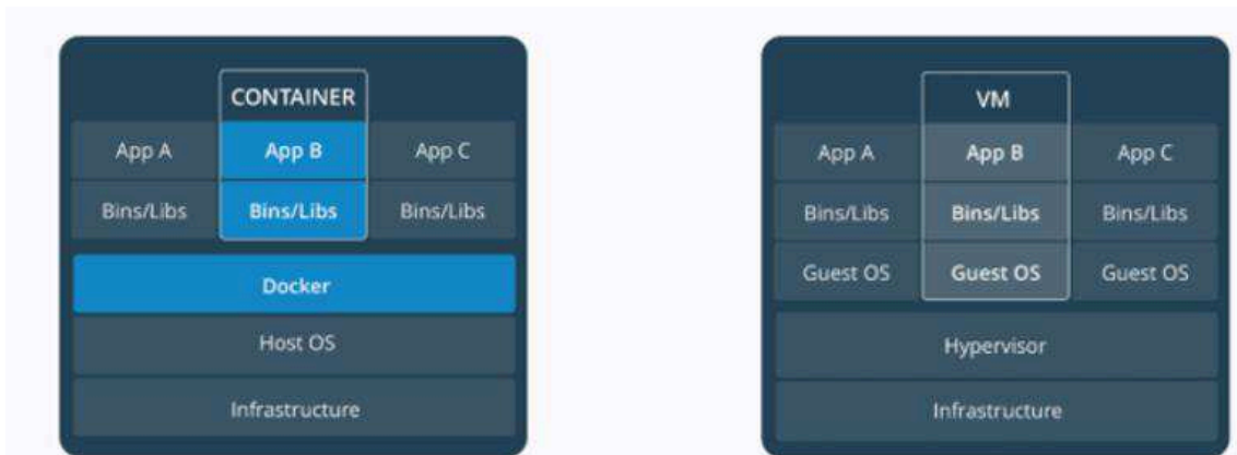
Figura 2. Comparação entre Docker (esquerda) e máquina virtual (direita)
