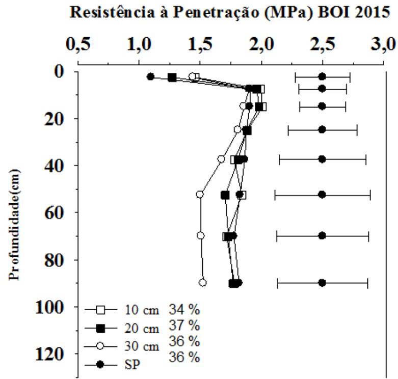
Figura 3. Resistência do solo à penetração (RP) na retirada dos animais, amostragem realizada em 14 de novembro de 2015, realizada até 0,8 m de profundidade, em diferentes alturas de pastejo: 0,10 m, 0,20 m, 0,30 m e SP (sem pastejo). Barras horizontais em cada profundidade indicam a diferença mínima significativa pelo teste de Tukey 5%.
