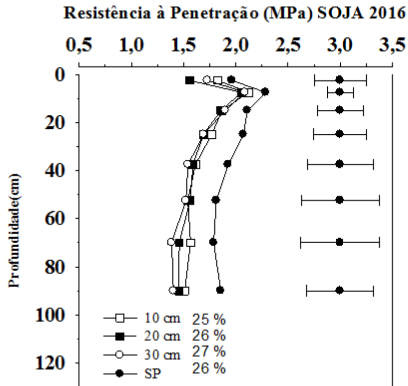
Figura 4. Resistência do solo à penetração (RP) após a colheita da cultura da soja, amostragem realizada em 18 de abril de 2016, realizada até 0,8 m de profundidade, em diferentes alturas de pastejo: 0,10 m, 0,20 m, 0,30 m e SP (sem pastejo). Barras horizontais em cada profundidade indicam a diferença mínima significativa pelo teste de Tukey 5% (DMS).
