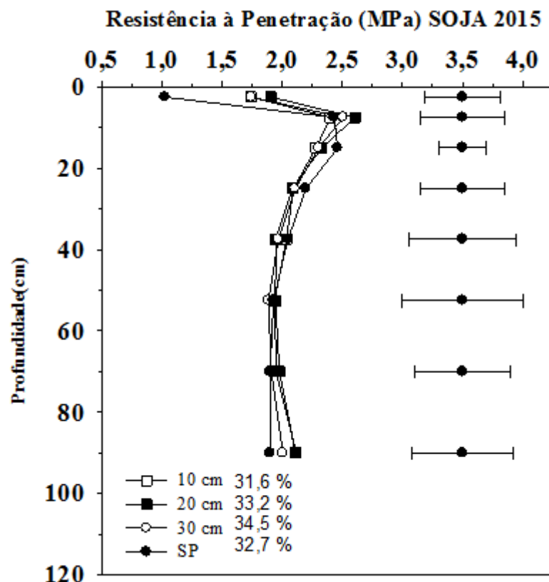
Figura 2. Resistência do solo à penetração (RP) na retirada da cultura da soja, amostragem realizada em 13 de maio de 2015, realizada até 0,8 m de profundidade, em diferentes alturas de pastejo: 0,10 m, 0,20 m, 0,30 m e SP (sem pastejo). Barras horizontais em cada profundidade indicam a diferença mínima significativa pelo teste de Tukey 5% (DMS).
