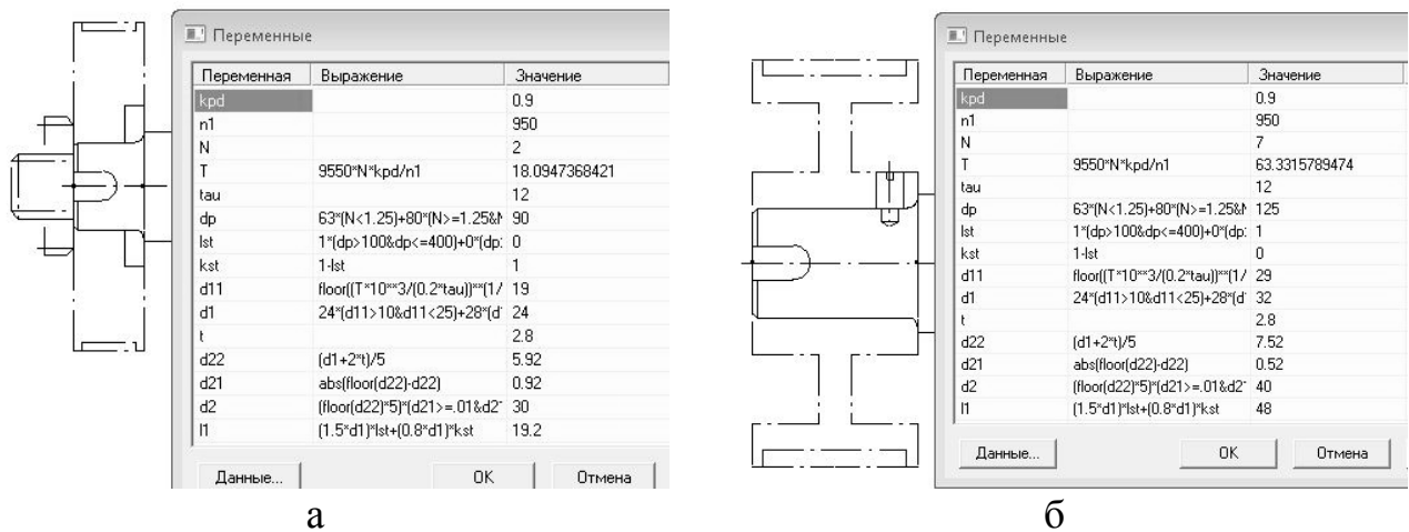
Рис.3. Варианты осевой фиксации: а – шкивы монолитной конструкции; б – шкивы дисковой конструкции
