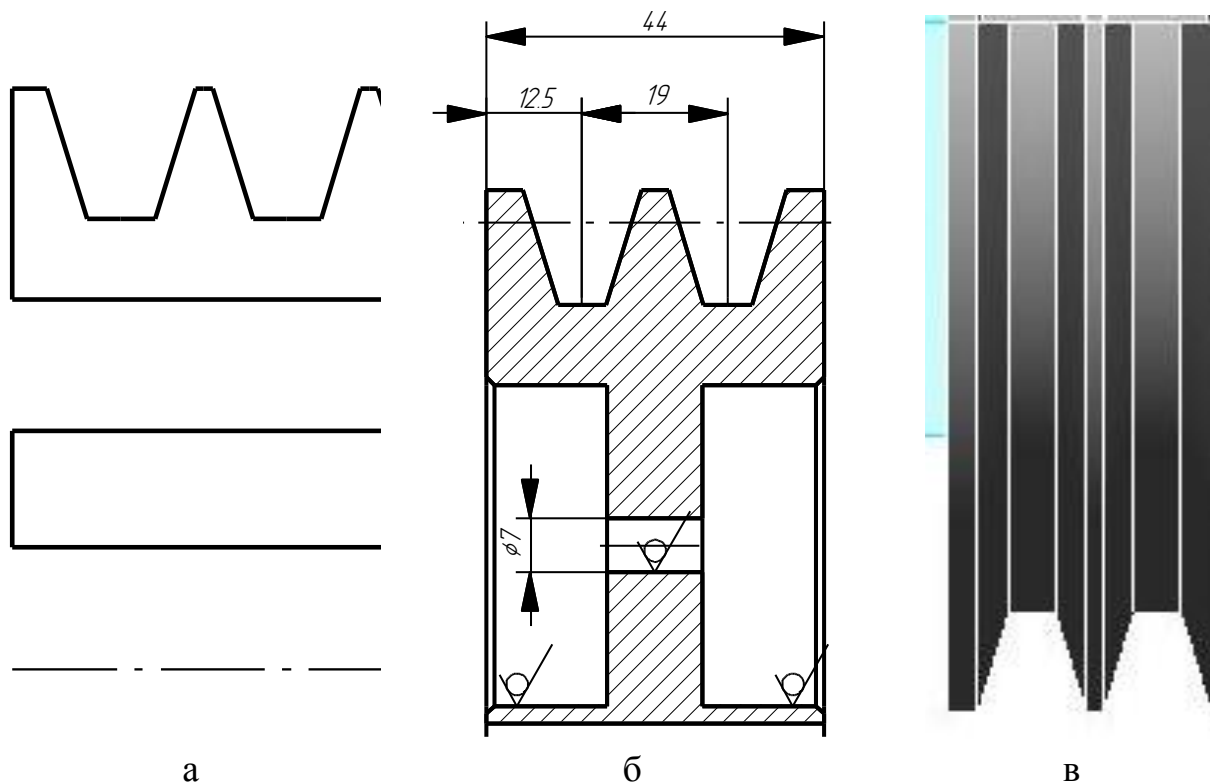
Рис.4. Шкив клиноременной передачи: а – фрагмент параметрической модели; б – фрагмент чертежа; в – фрагмент 3D – модели
