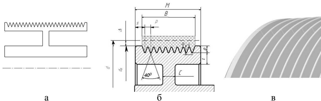
Рис.5. Шкив поликлиновой передачи: а – фрагмент параметрической модели; б – фрагмент чертежа; в – фрагмент 3D – модели
