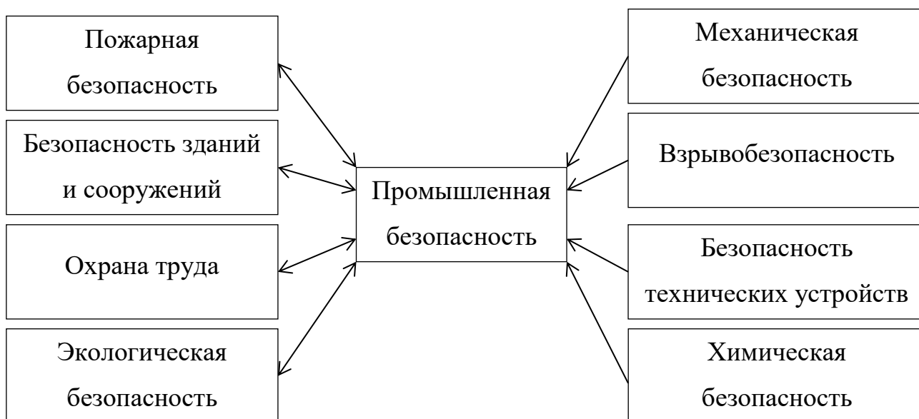
Рисунок 2 – Виды безопасности
