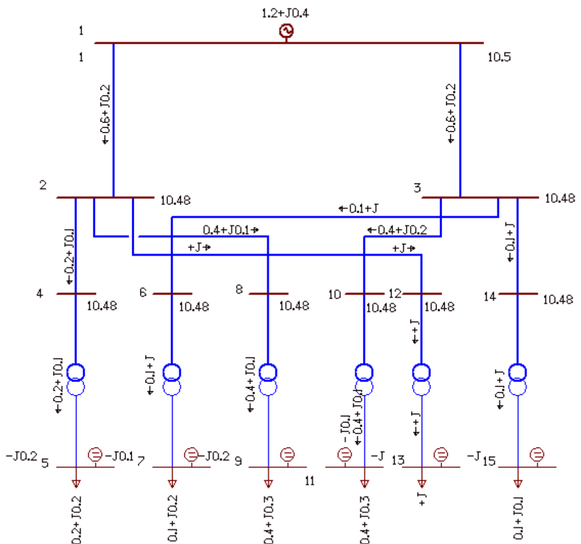
Рисунок 29 – Цифровая расчетная модель ЭЭС с установкой КУ на шинах 0,4кВ
