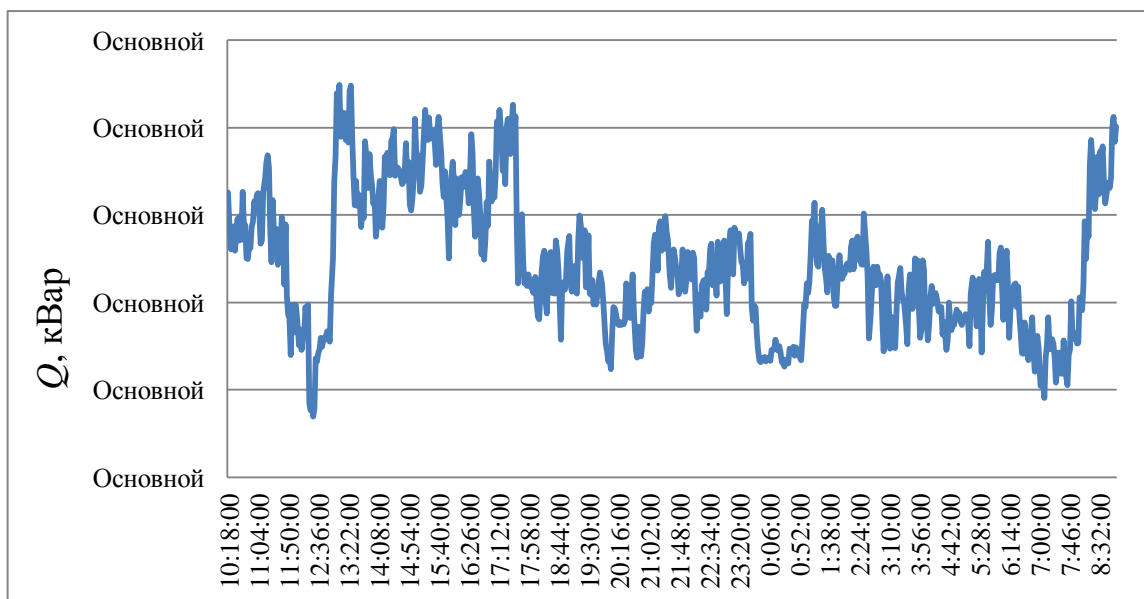
Рисунок 4 – Суточный график реактивной мощности ТП1 ввод1
