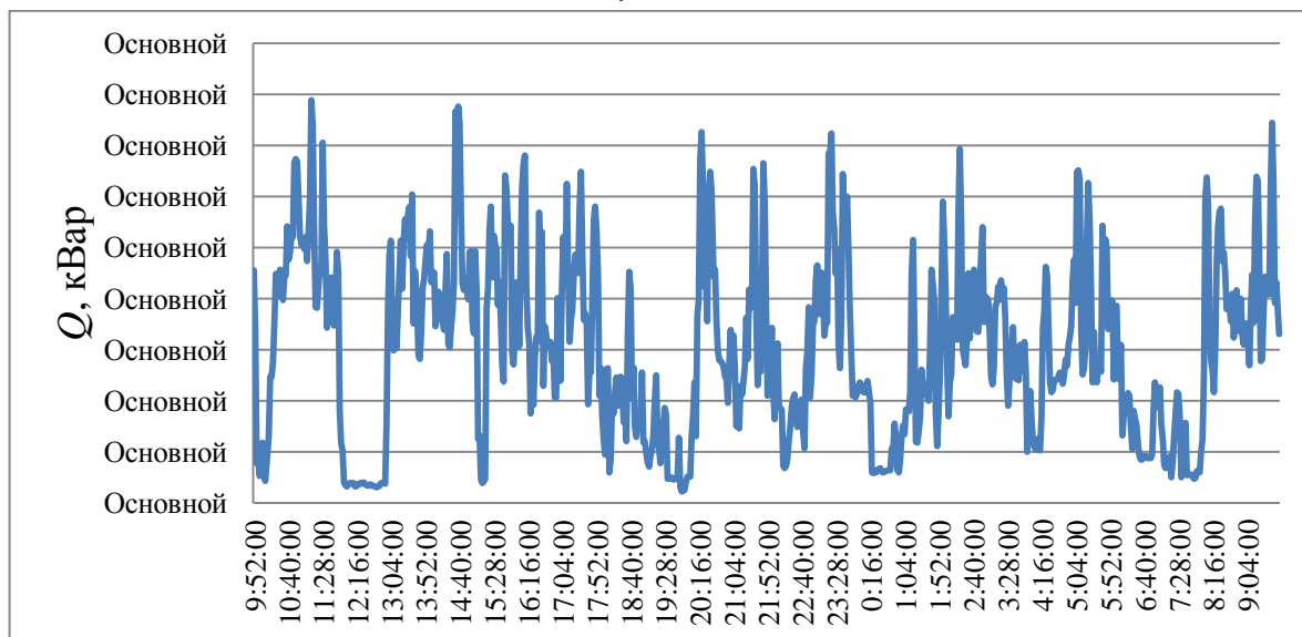
Рисунок 5 – Суточный график реактивной мощности ТП1 ввод2
