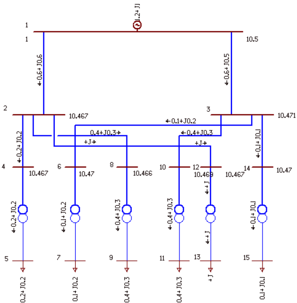
Рисунок 23 – Цифровая расчетная модель ЭЭС
