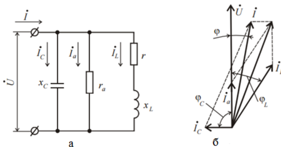
Рисунок 1 – Нагрузка в цепи переменного тока и ее векторная диаграмма:
