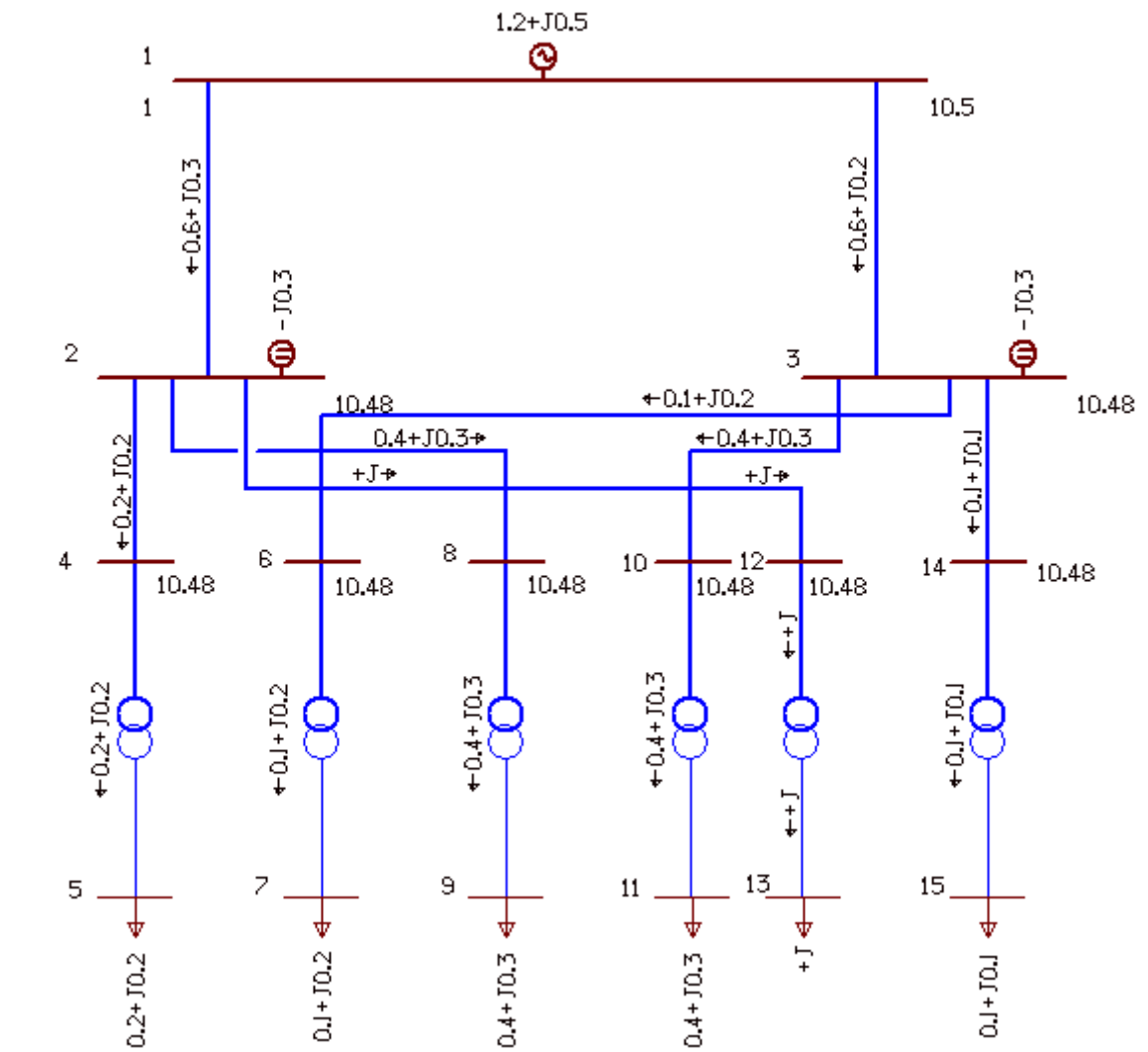
Рисунок 26 – Цифровая расчетная модель ЭЭС с установкой КУ на шинах 10кВ
