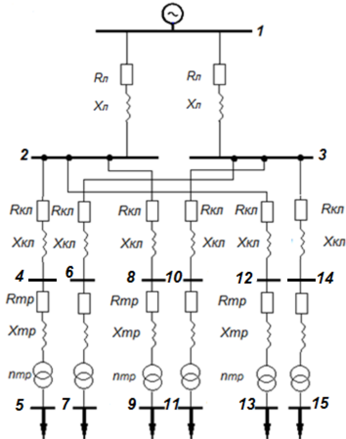
Рисунок 20 – Схема замещения
