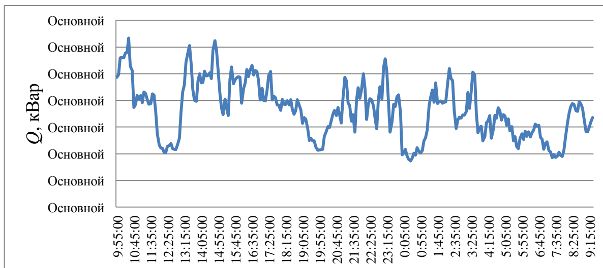
Рисунок 6 – Суточный график реактивной мощности ТП2 ввод1
