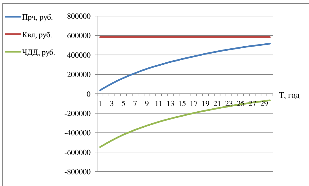
Рисунок 25 – Дисконтированные показатели экономической эффективности внедрения конденсаторных установок напряжением 10кВ
