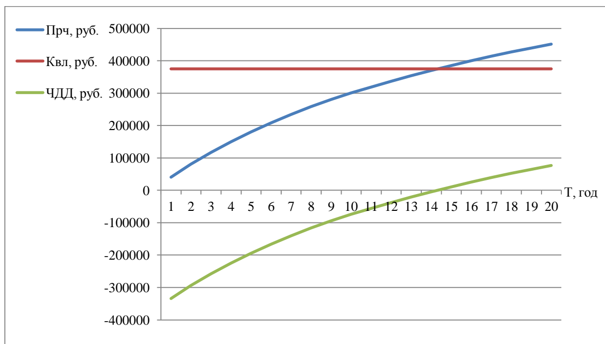
Рисунок 26 – Дисконтированные показатели экономической эффективности внедрения конденсаторных установок напряжением 0,4кВ
