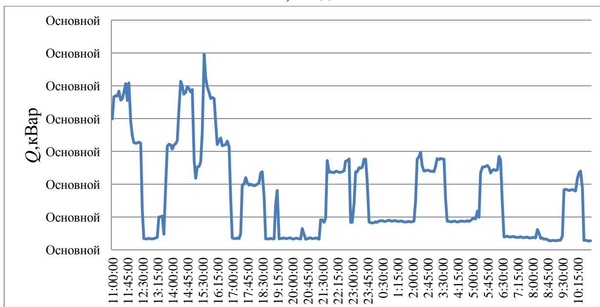
Рисунок 9 – Суточный график реактивной мощности ТПЗ ввод2
