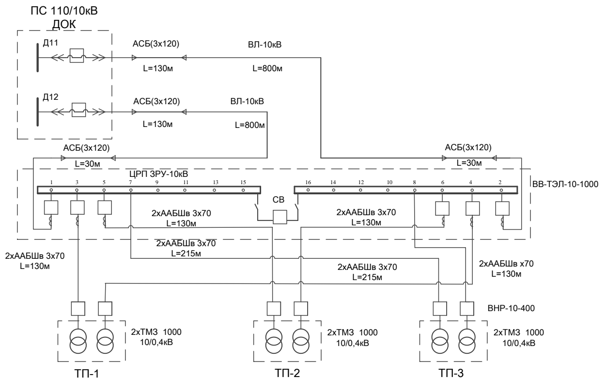
Рисунок 3 – Однолинейная схема электроснабжения ООО «ЗКПД ТДСК» площадка №2
