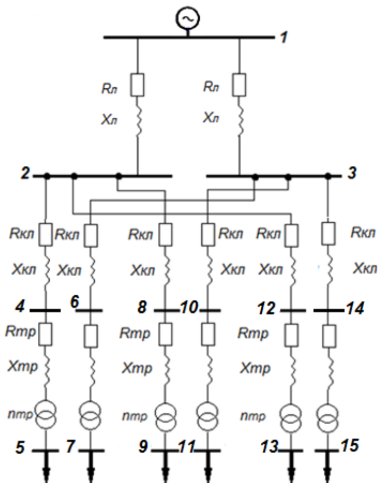
Рисунок 10 – Схема замещения ООО «ЗКПД ТДСК» площадка №2
