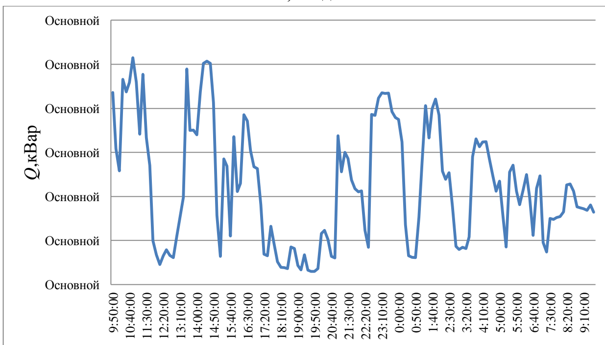
Рисунок 7 – Суточный график реактивной мощности ТП2 ввод2
