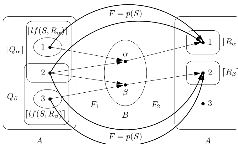
15.8. ábra. Ellenpélda
