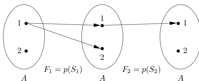
15.10. ábra. Ellenpélda
