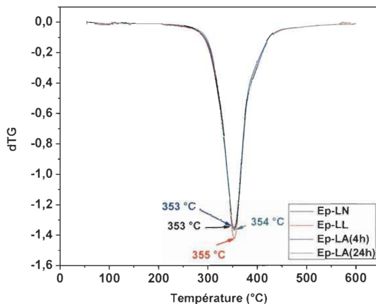
Figure III.56 Courbes DTG des composites lin/époxy.
