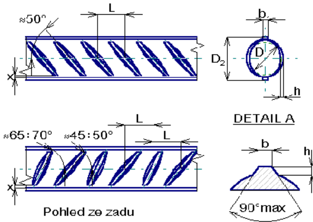
Obr.č.5 – tvar prutů oceli 10 505 R [15]
