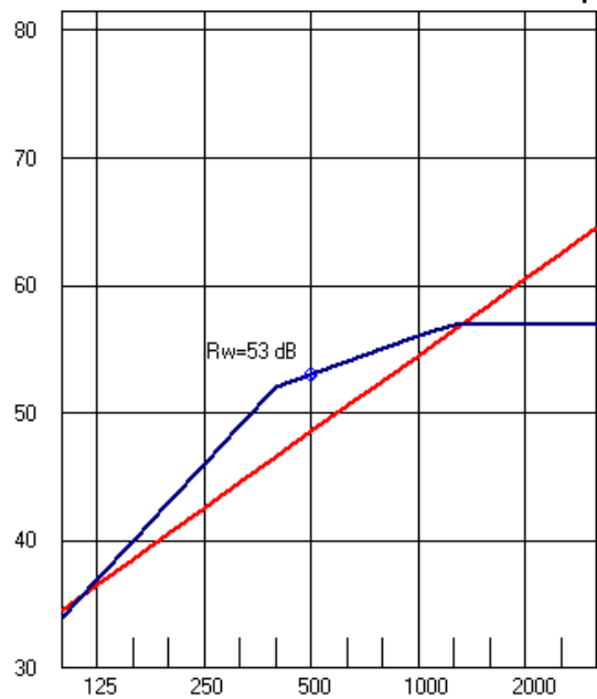
Graf (laboratorní) neprůzvučnosti R Obvodová konstrukce - vzduchová neprůzvu
