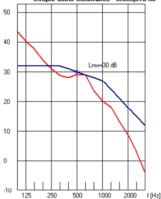
Graf norm. hladiny kročej. zvuku Stropní dělicí konstrukce - kročejová ne
