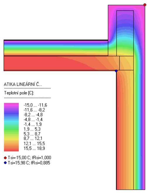
Obr. č. 3 Pole teplot oblast atiky
