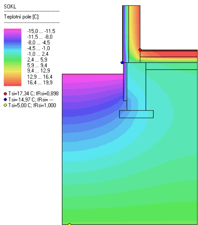
Obr. č. 2 Pole teplot oblast soklu
