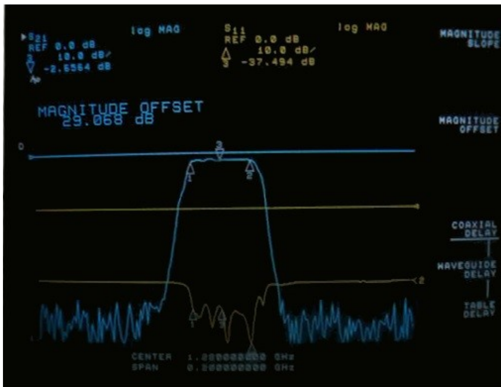
Obr. 8: Kmitočtový průběh filtru s osmnácti rezonátory
