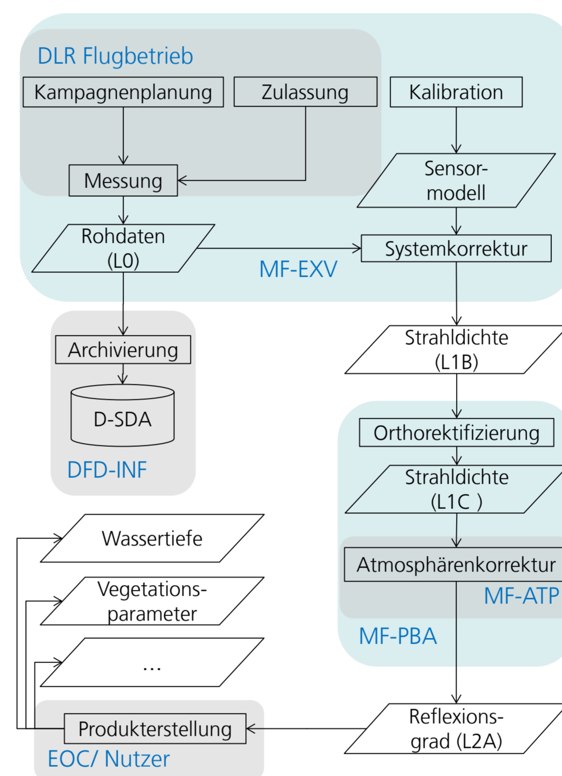
Abb. 4: Ablaufdiagramm der flugzeuggestützten Fernerkundung durch OpAIRS (blau hinterlegt) mit Unterstützung verschiedener EOC Abteilungen (grau hinterlegt)
