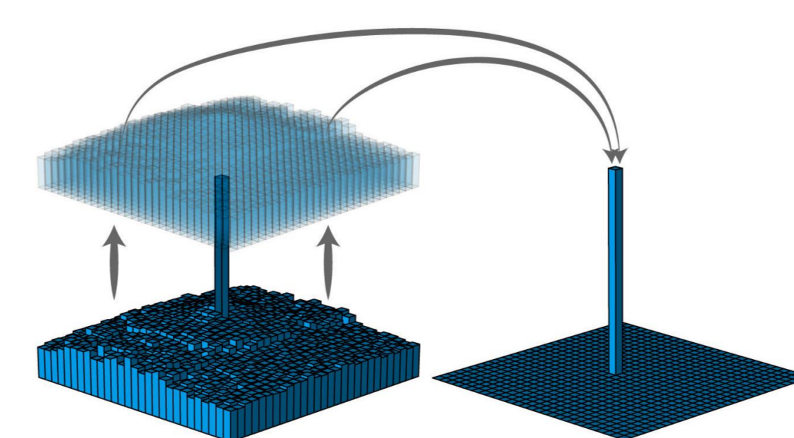
Abb. 6: Streulichtkorrektur im idealisierten Fall monochromatischer Beleuchtung eines einzigen Pixels. Falsch registrierte Beiträge anderer Detektorpixel werden dem korrekten Pixel/Kanal zugeordnet. (Bild: J. Brachmann, DLR Oberpfaffenhofen)
