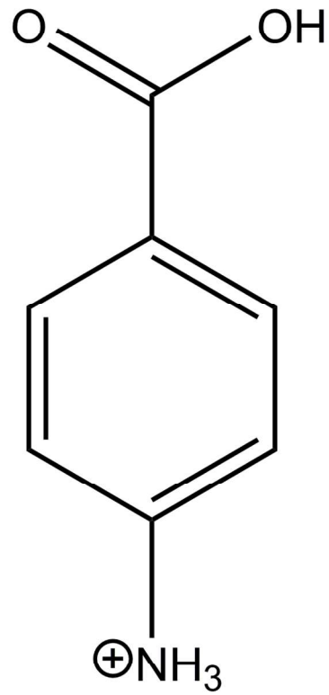
PABA-NH 3 +
