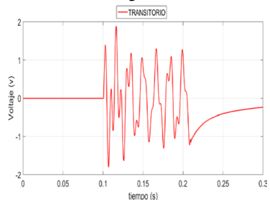
(a). Fenómeno transitorio originado.
