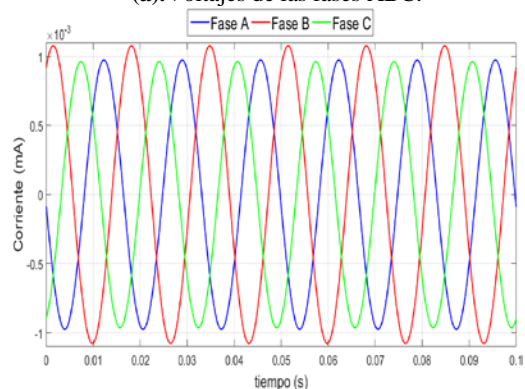
(b). Corrientes de las fases ABC.
