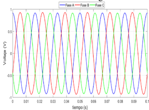
(a). Voltajes de las fases ABC.
