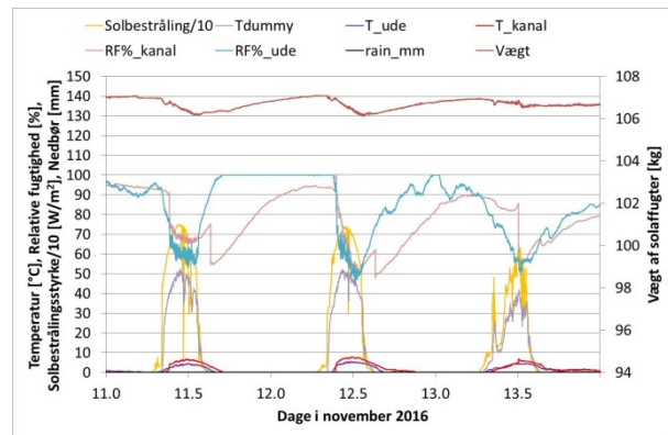
Figur 11. Måleresultater. Luftflow i alle nattetimer mens luftflow i dagtimer starter når T_{dummy,start} > 60^{\circ}\text{C} og stopper når T_{dummy,stop} < 50^{\circ}\text{C} .
