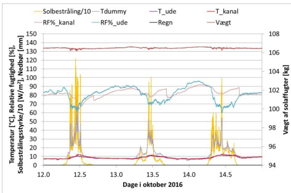
Figur 11. Måleresultater. Luftflow i alle nattetimer mens luftflow i dagtimer starter når T_{dummy,start} > 60^{\circ}\text{C} og stopper når T_{dummy,stop} < 50^{\circ}\text{C} .
