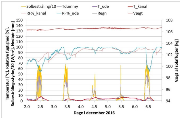
Figur 12. Måleresultater. Luftflow i alle nattetimer mens luftflow i dagtimer starter når T_{dummy,start} > 60^{\circ}\text{C} og stopper når T_{dummy,stop} < 50^{\circ}\text{C} (til venstre) og luftflow i dagtimer starter når T_{dummy,start} > 40^{\circ}\text{C} og stopper når T_{dummy,stop} < 30^{\circ}\text{C} (til højre).
