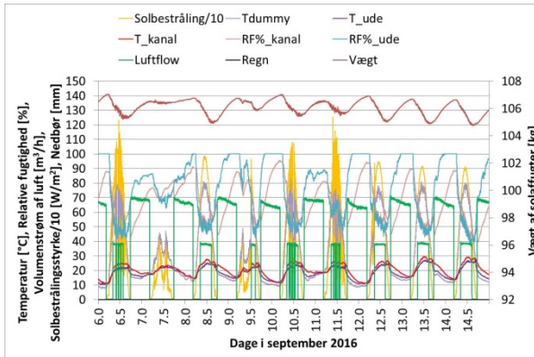
Figur 9. Måleresultater. Luftflow i alle nattetimer mens luftflow i dagtimer starter når T_{dummy,start} > 60^{\circ}C og stopper når T_{dummy,stop} < 50^{\circ}C .
