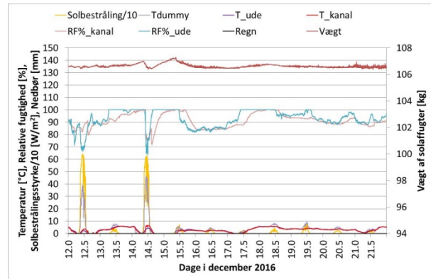
Figur 12. Måleresultater. Luftflow i alle nattetimer mens luftflow i dagtimer starter når T_{dummy,start} > 60^{\circ}\text{C} og stopper når T_{dummy,stop} < 50^{\circ}\text{C} (til venstre) og luftflow i dagtimer starter når T_{dummy,start} > 40^{\circ}\text{C} og stopper når T_{dummy,stop} < 30^{\circ}\text{C} (til højre).
