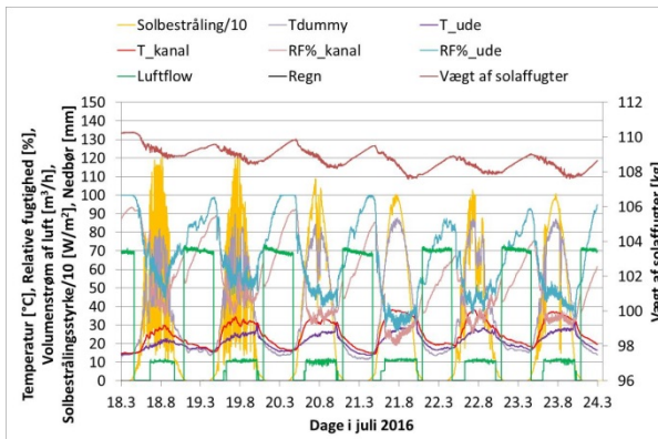
Figur 8. Måleresultater. Til venstre: Luftflow i alle dag- og nattetimer. Til højre: Luftflow i alle nattetimer mens luftflow i dagtimer starter når T_{dummy,start} > 60^{\circ}C og stopper når T_{dummy,stop} < 35^{\circ}C .
