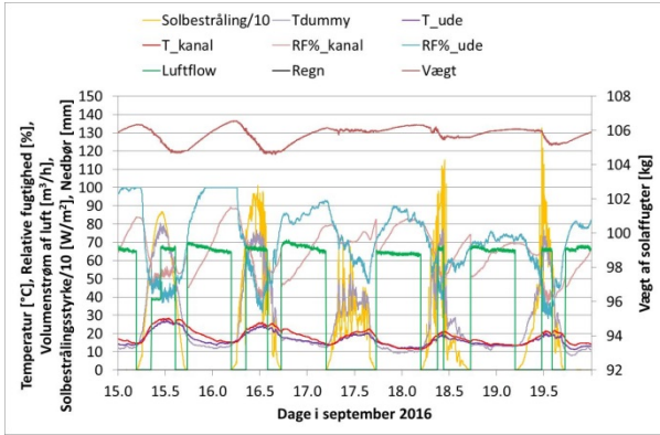
Figur 10. Måleresultater. Luftflow i alle nattetimer mens luftflow i dagtimer starter når T_{dummy,start} > 60^{\circ}\text{C} og stopper når T_{dummy,stop} < 50^{\circ}\text{C} .
