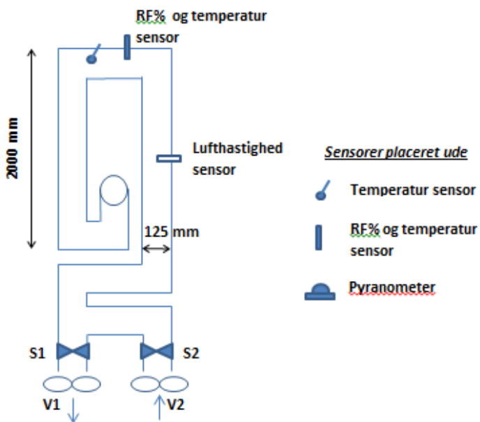
Figur 3. Principskitse af prøvestanden
