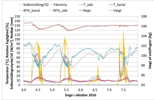
Figur 10. Måleresultater. Luftflow i alle nattetimer mens luftflow i dagtimer starter når T_{dummy,start} > 60^{\circ}\text{C} og stopper når T_{dummy,stop} < 50^{\circ}\text{C} .
