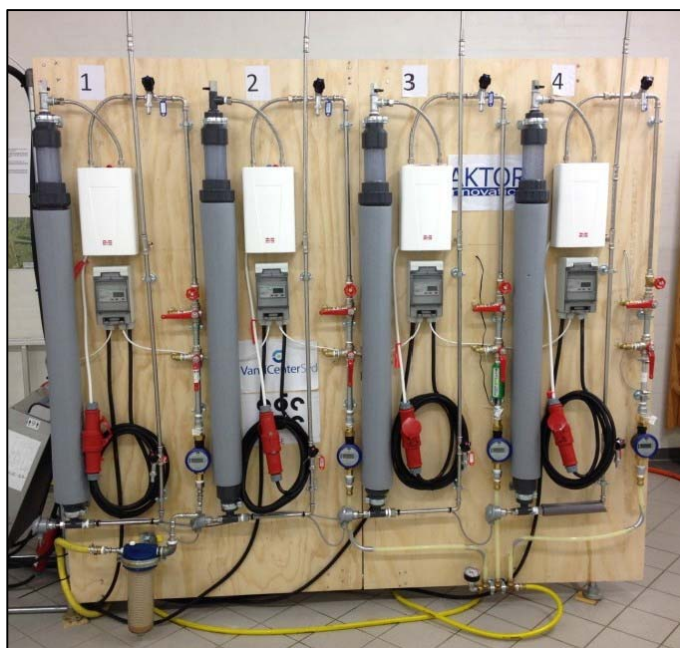
Figur 17 Opstilling af fire parallelle forsøgslinjer på Dalumværket.
