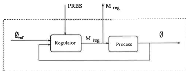
Figur 11. Slutna systemet
