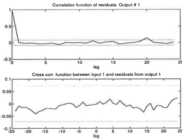
Figur 8: Ordning 4 (80 Hz). I figuren är 99%-iga konfidensintervall markerade.
