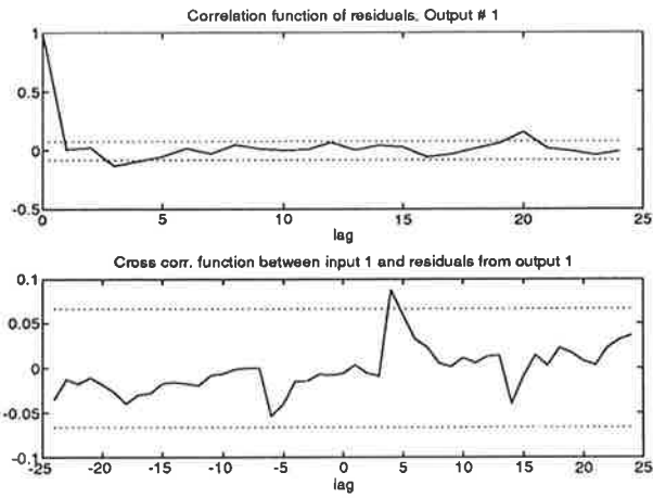
Figur 6: Ordning 2 (80 Hz). I figuren är 99%-iga konfidensintervall markerade.
