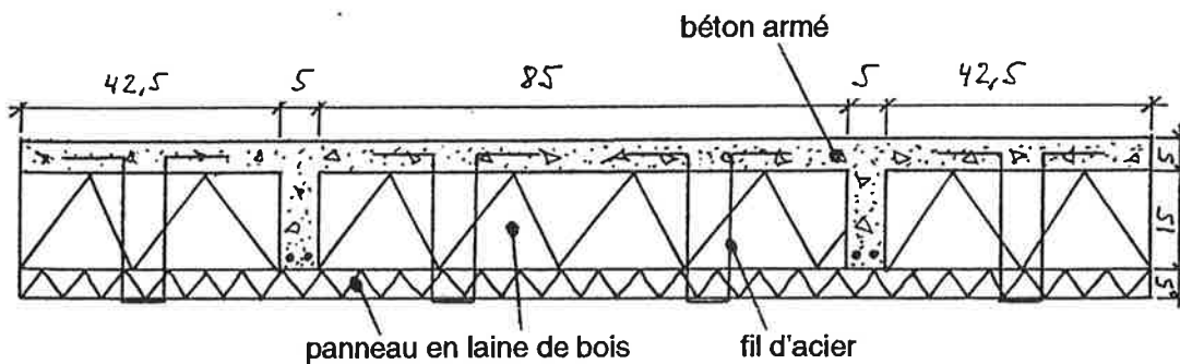
Figure 4.2.3. Toiture avec ossature porteuse en béton et isolation thermique avec panneaux en laine de bois. Les ponts thermiques sont interrompus par une suite ininterrompue de panneaux en laine de bois.
