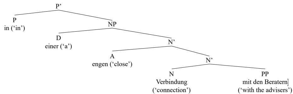
Figure 13.2: The structure of the PP in einer engen Verbindung mit den Beratern ('in a close connection with the advisers')
