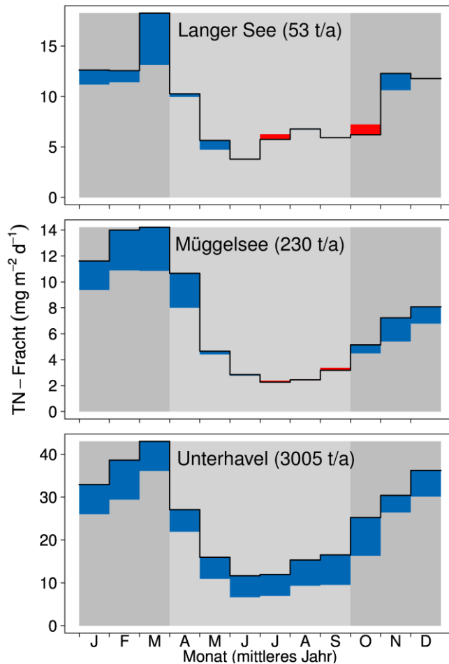
Abbildung 26 Saisonale Dynamik der TN-Frachten und Nettoexport (rot) bzw. NettoRetention (blau) für den Langer See, den Müggelsee und die Unterhavel als Mittelwert der Untersuchungsjahre 2000 - 2010 (Jahresfracht von TN für die einzelnen Gewässer in Klammern)
