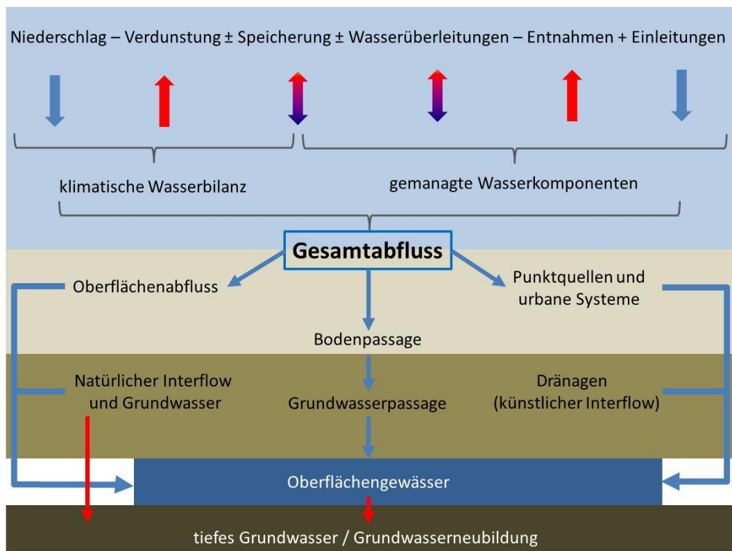
Abbildung 1 Schematische Darstellung der für MONERIS verwendeten Wasserhaushaltskomponenten und deren Aufteilung in die unterschiedlichen Abflusskomponenten
