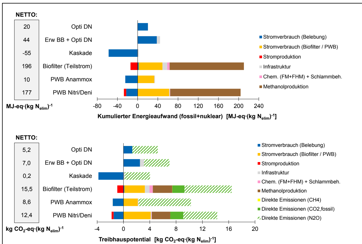
Abbildung 9 KEA und THP der Szenarien im Vergleich pro kg eliminiertem Stickstoff
