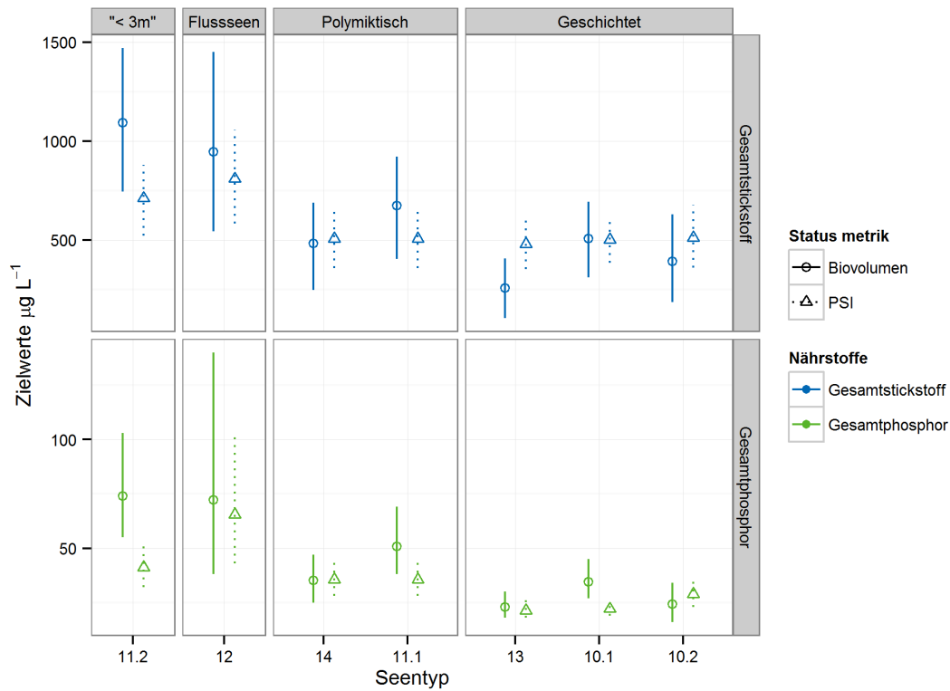
Abbildung 6 TN- und TP-Zielwerte basierend auf Phytoplanktonbiovolumen und PSI.
