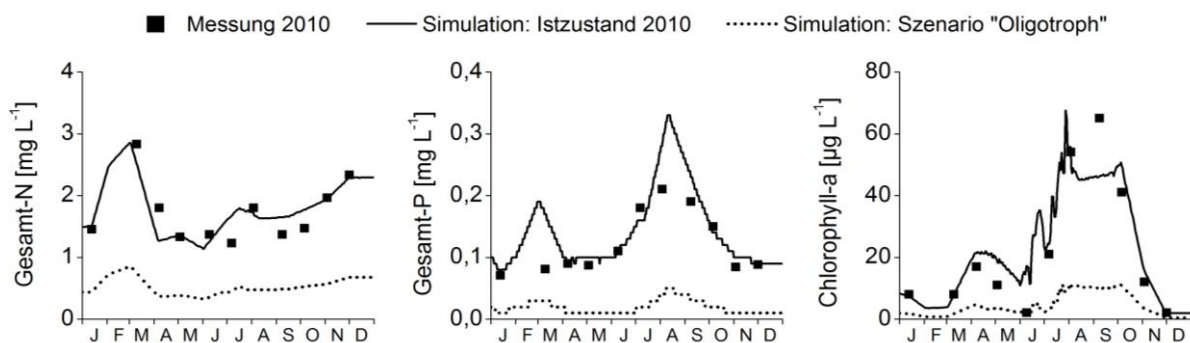
Abbildung 13 Für den Istzustand 2010 gemessene und simulierte Konzentration von TN-, TP- und Chlorophyll-a in der Berliner Stadtspre bei km 8 des simulierten Flussabschnitts. Die gepunktete Linie zeigt die Simulationsergebnisse für einen hypothetisch oligotrophen Gewässerzustand (Szenario „Oligotroph“).
