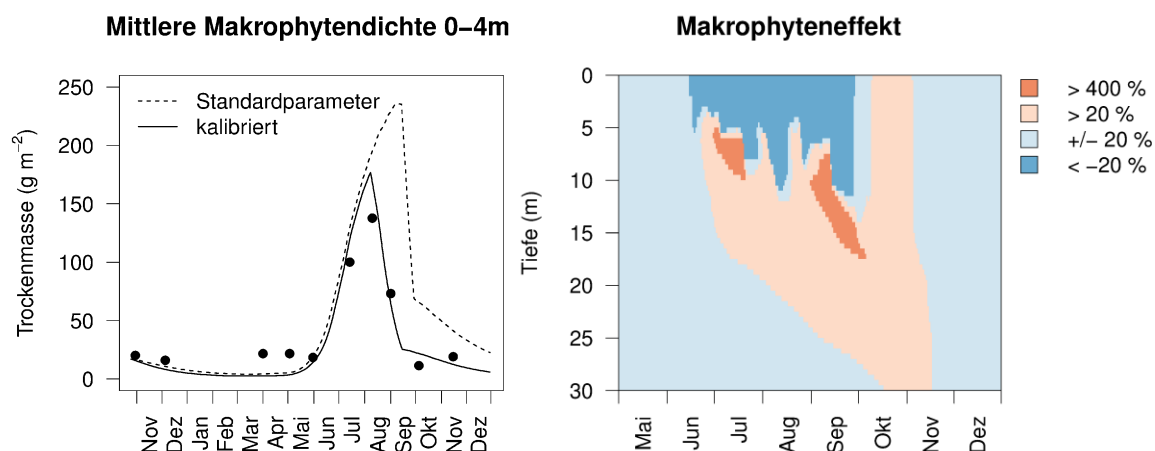
Abbildung 7 Simulierte mittlere Makrophytenbiomasse in 0 m bis 4 m Tiefe unter Anwendung der Standardparameter und mit für die Hauptarten des Scharmützelsees kalibrierten Parametern (links, Daten: Marlene Pätzig, BTU Cottbus) und simulierter Makrophyteneffekt auf das Gesamtphytoplankton (rechts). Der Makrophyteneffekt ( ME = (X - X_{Mac})/X ) ist die relative Differenz der Szenarien mit
