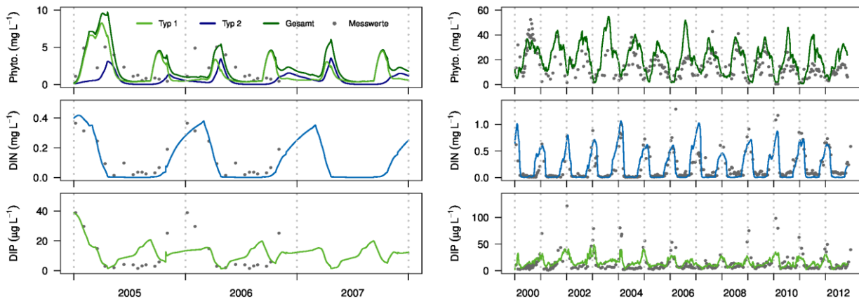
Abbildung 6 Referenzszenario für den Scharmützelsee (links, Zweischicht-Modell) und für den Langen See (rechts, Einschichtmodell); Symbole: Messwerte, durchgezogene Linien: Modellsimulation. Typgruppe 1: schnell wachsendes Phytoplankton, Typgruppe 2: langsam wachsendes Phytoplankton einschließlich N 2 -Fixierer, gelöster anorganischer Stickstoff (DIN) und Phosphor (DIP).
