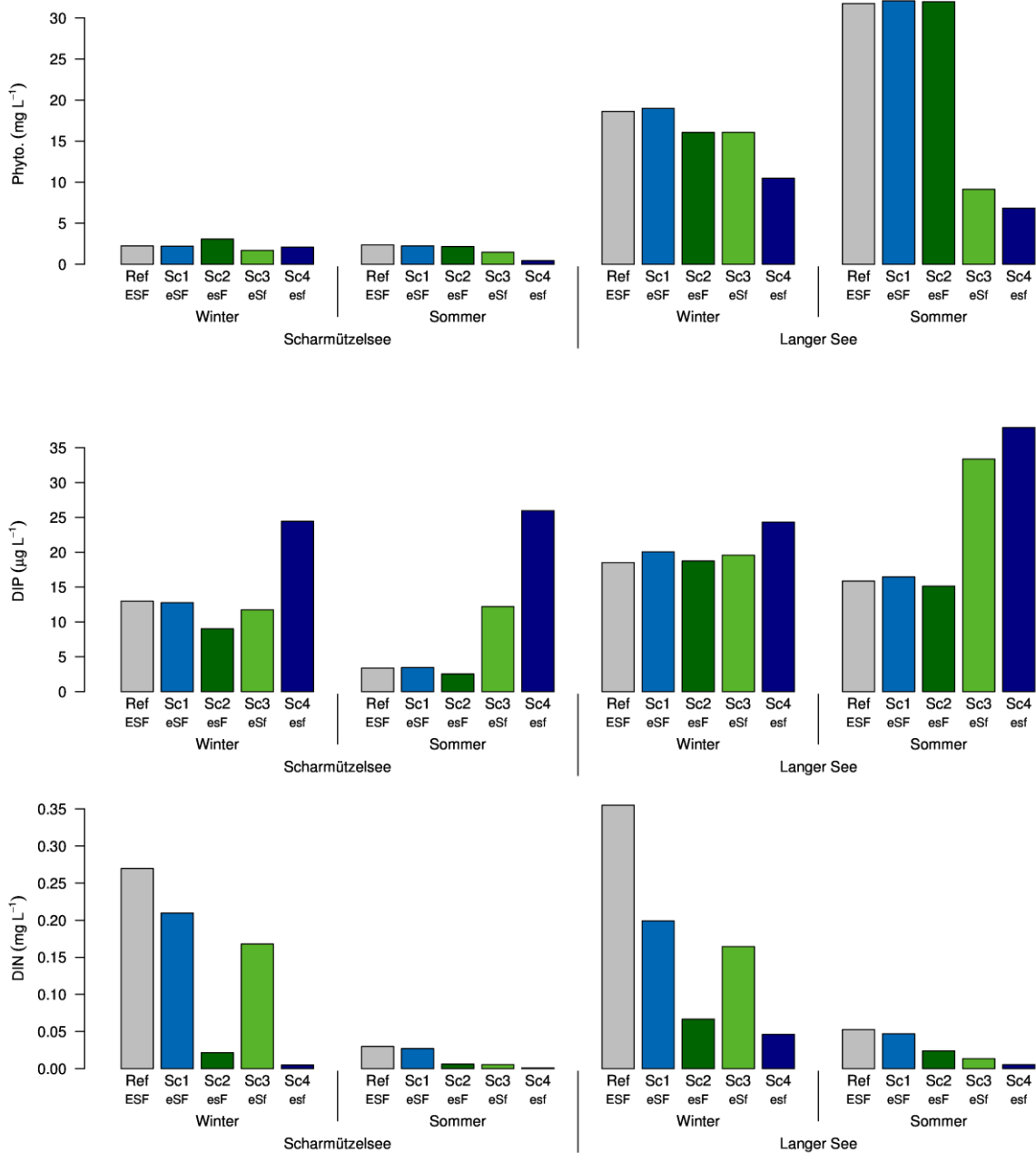
Abbildung 10 Mittelwerte von Phytoplankton, gelöstem anorganischen Phosphat (DIP) und gelöstem anorganischen Stickstoff im 2. Simulationsjahr für die Winter- (Dezember - April) bzw. Sommerperiode (Mai - Oktober). Die Szenarien definieren sich wie folgt: externer Stickstoffeintrag 100 % („E“) bzw. 50 % („e“) hohe („S“) bzw. niedrige („s“) N-Freisetzung aus dem Sediment, mit bzw. ohne N 2 -fixierende Cyanobakterien („F“ bzw. „f“).
