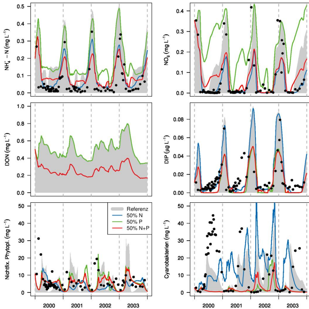
Abbildung 11 Simulationen mit dem detaillierten Stickstoffumsatzmodell DNSmod für den Langen See. Symbole: gemessene Daten (Frischmasse), Referenzszenario grau schattiert, Szenario mit 50 % N (blau) bzw. 50 % P-Reduktion (grün) sowie simultaner N- und P-Reduktion (rot). Bei den Vergleichsdaten des Phytoplanktons ist zu beachten, dass nicht alle der zum Vergleich herangezogenen Cyanobakterien (rechts unten) N 2 -Fixierer sind.
