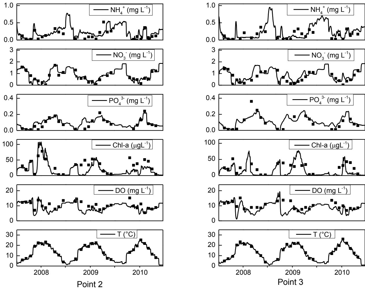
Abbildung 17 Ergebnisse der Gewässergütemodellierung für die Untere Havel. Die durchgezogene Linie zeigt die Simulationsergebnisse, Punkte die Messwerte. Links UHV-km 7,5 (point 2), rechts UHV-km 11,0 (point 3).
