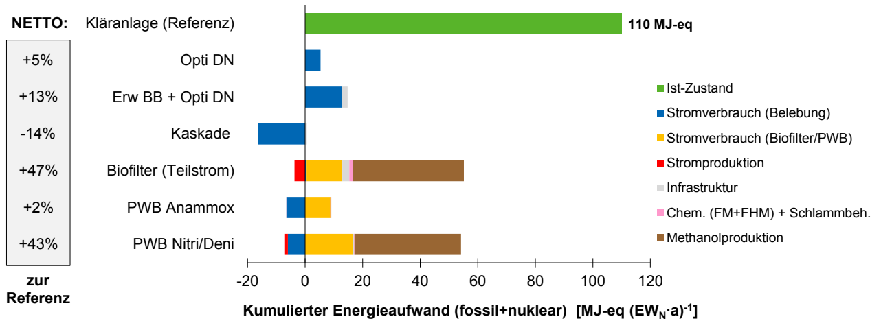
Abbildung 7 Kumulierter Energieaufwand der Szenarien verglichen zur Referenz
