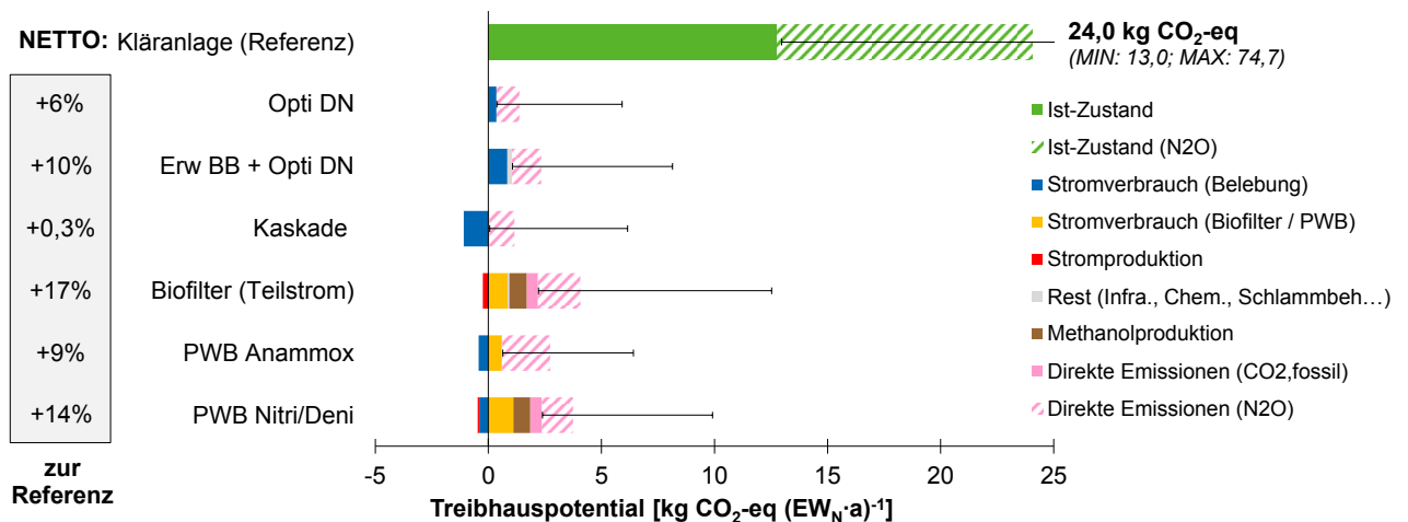
Abbildung 8 Treibhauspotential der Szenarien verglichen zum Referenzzustand inklusive Unsicherheiten in den direkten N 2 O-Emissionen aus der biologischen N-Reduktion
