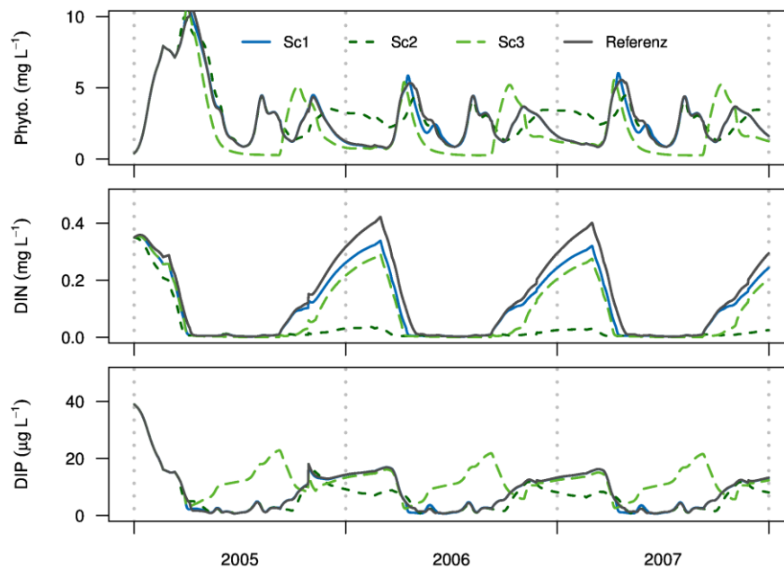
Abbildung 8 N-Reduktionsszenarien für den Scharmützelsee; gelöster anorganischer Phosphor (DIP), gelöster anorganischer Stickstoff (DIN) und Gesamtphytoplankton für die durchmischte Schicht. Szenario 1: externe N-Belastung auf 50 % reduziert; Szenario 2: externe N-Belastung auf 50 % und interne N-Belastung maximal reduziert, Szenario 3: externe N-Belastung 50 % reduziert, keine N_2 -Fixierer.
