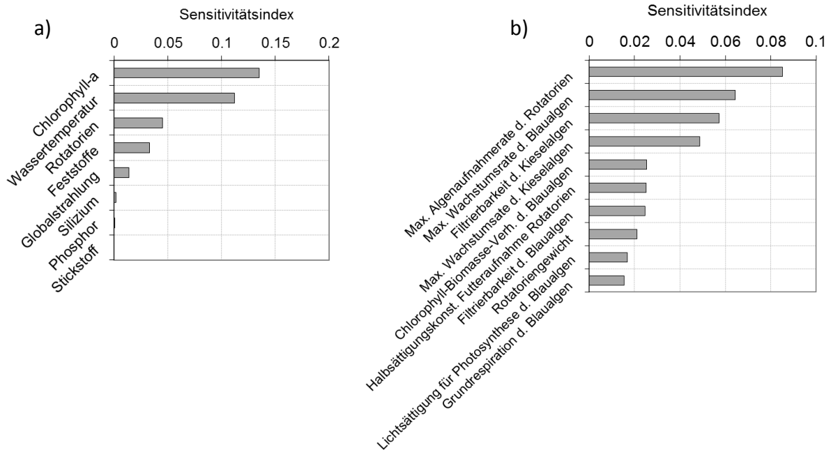
Abbildung 14 Sensitivität von Chlorophyll-a bezüglich der einflussreichsten Zustandsvariablen (a) und Modellparameter (b) für den simulierte Istzustand 2010 der Berliner Stadtspreet.
