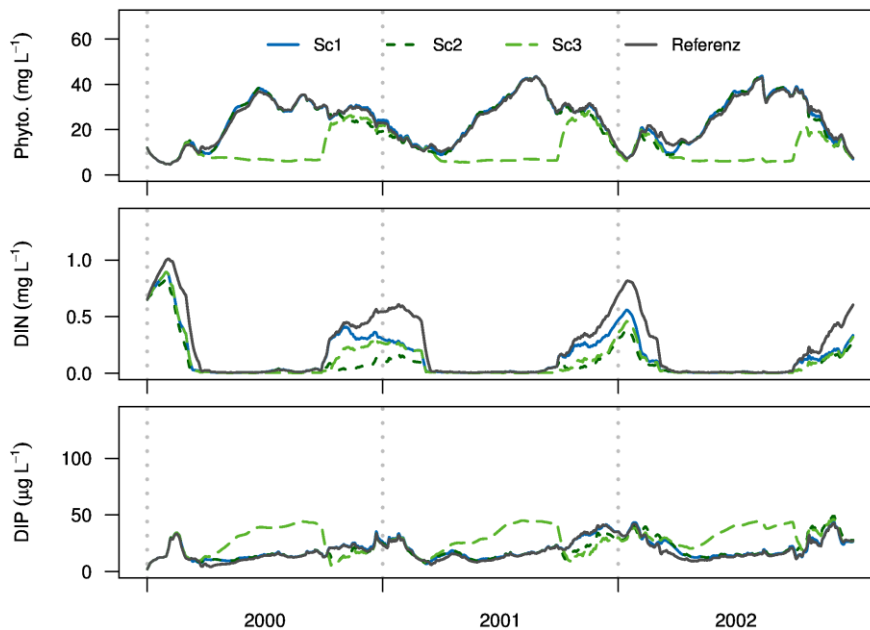
Abbildung 9 N-Reduktionsszenarien für den Langen See (Szenarien wie Abbildung 8).
