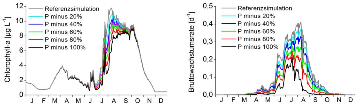
Abbildung 16 Für einen hypothetisch oligotrophen Zustand der Berliner Stadtspreie simulierte Chlorophyll-a-Konzentration und Bruttowachstumsrate des Phytoplanktons bei unterschiedlichen P-Eingangskonzentrationen (Szenario „Oligotroph“).
