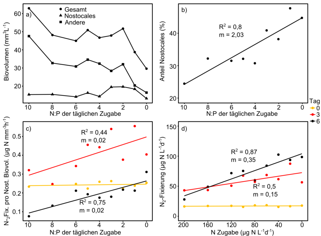
Abbildung 27 a) Zusammenhang des Biovolumens mit dem N:P Verhältnis der täglichen Zugabe, b) Zusammenhang des Anteils der Nostocales (Tag 6) am Biovolumen mit dem N:P Verhältnis der täglichen Zugabe und c) Zusammenhang der N_2 -Fixierung pro Nostocalem Biovolumen mit dem N:P Verhältnis der täglichen Zugabe. d) Absolute N_2 -Fixierung in Abhängigkeit der täglich zugegebenen Stickstoffmenge. R^2 : Bestimmtheitsmaß der Regression, m: Steigung der Regression.
