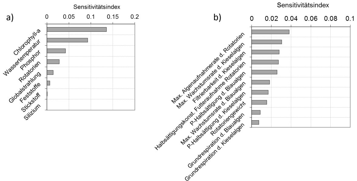
Abbildung 15 Sensitivität von Chlorophyll-a bezüglich der einflussreichsten Zustandsvariablen (a) und Modellparameter (b) für den hypothetisch oligotrophen Zustand der Berliner Stadtspreet (Szenario „Oligotroph“)
