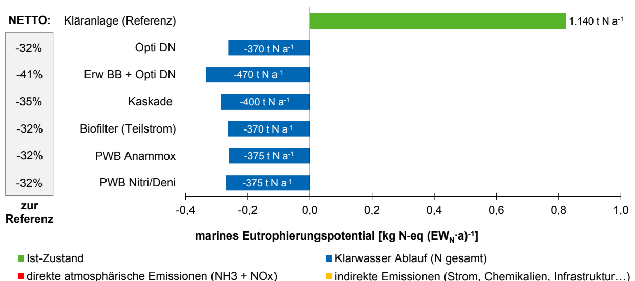
Abbildung 6 Marines Eutrophierungspotential (N-Emissionen) der Szenarien verglichen zur Referenz
