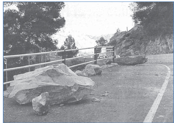
FIGURA 2. Foto de los desprendimientos sobre la carretera RM-520 (km 6); producidos por el terremoto de Mula (5.2 M. 2/2/1999). Periódico La Verdad.
